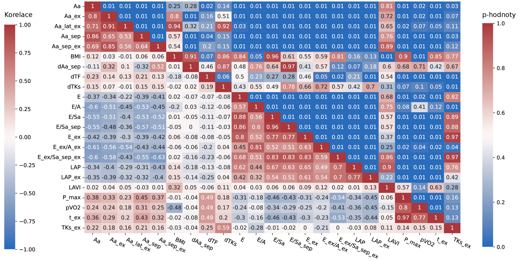
Obr. A.3: Korelační matice signifikantních příznaků
