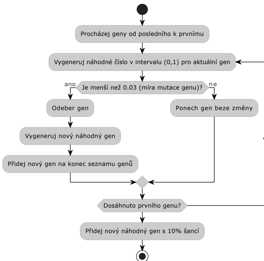
Obrázek 5.5: Diagram aktivit metody MutateGenes , která je operátorem mutace v rámci genů rostliny. Metoda zamění některé geny v nové rostlině za jiné náhodné.
