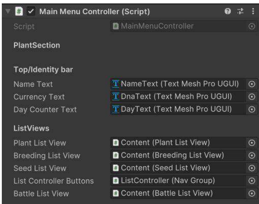
Obrázek 5.6: MainMenuController využívá reference na zobrazovací komponenty, které ukládá dle sekce, ke které komponenta spadá. Skript je vizualizován v Unity Inspectoru.
