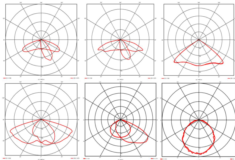
Obr. 4: Příklady křivek svítivosti (1,2 - LED svítidla veřejného osvětlení; 3,4 - LED parková svítidla; 5 - LED reflektor; 6 - interiérové LED svítidlo)
