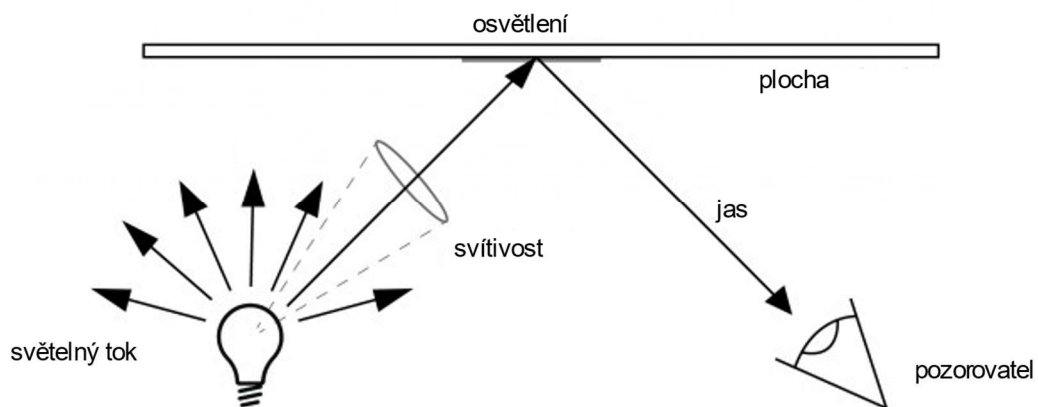
Obr. 5: Vzájemný vztah světelného toku, svítivosti, osvětlení a jasu
