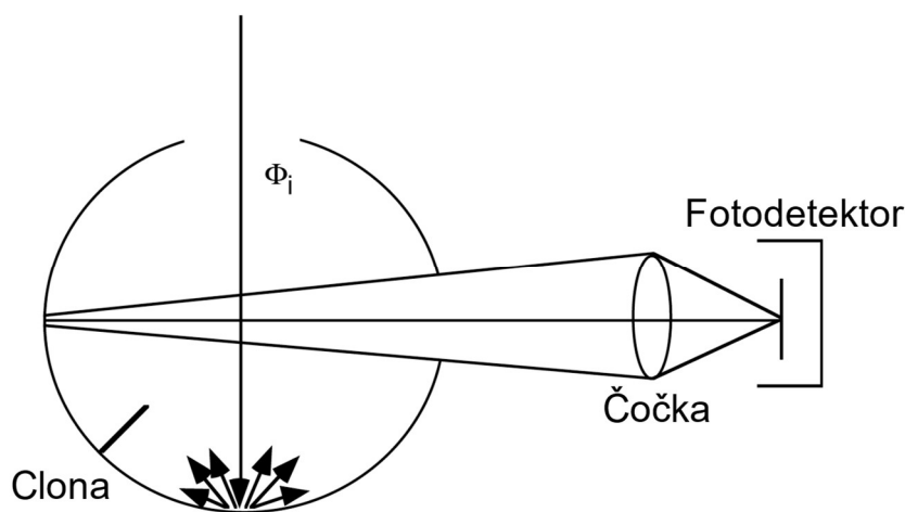
Obr. 18: Příklad optického systému kulového integrátoru s externí čočkou a fotodetektozem
