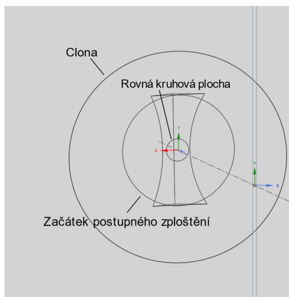
Obr. 32: Provedení zploštění stěny 1. polokoule – pohled zezadu, drátový model
