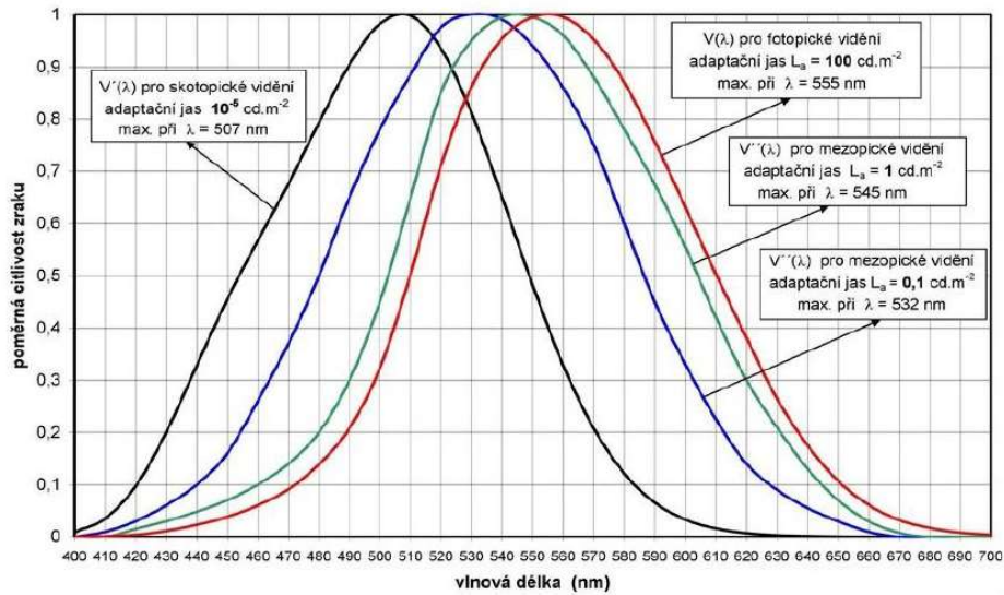
Obr. 1: Průběhy poměrné spektrální světelné účinnosti záření pro různé adaptační jasy L_a [1]
