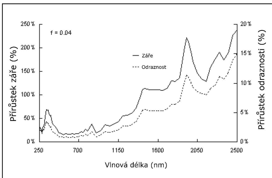
Obr. 17: Graf závislosti poměrného nárůstu záře a odraznosti na vlnové délce [7, upraveno]
