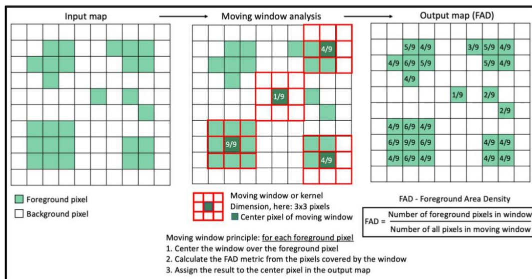
Obr. 27: Princip výpočtu FAD-MS: pohyblivé okno velikosti n x n (zde 3x3) je umístěno nad daným pixelem v popředí, je vypočítána metrika a výsledná hodnota je přiřazena na stejné místo na výstupní mapě. Centrální panel ukazuje čtyři příkladové lokace pro ilustraci procesu
