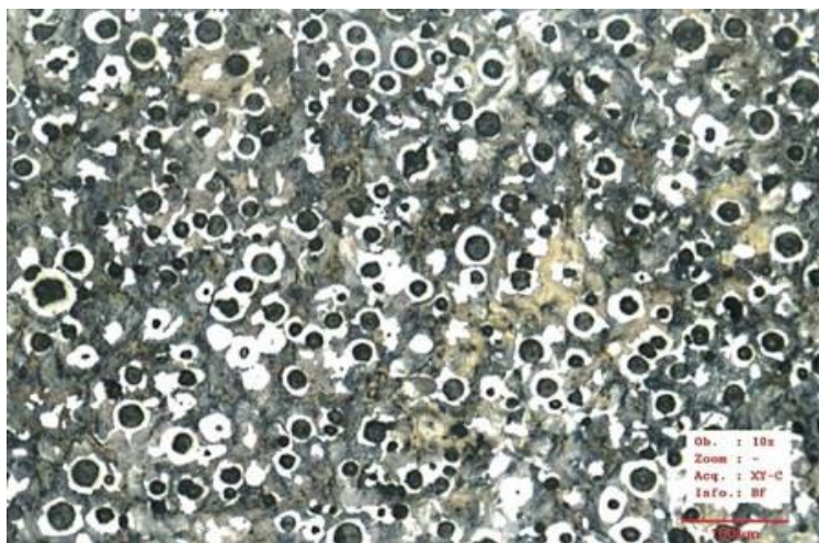
Obr. 2.13 Struktura tvárné litiny pod mikroskopem
