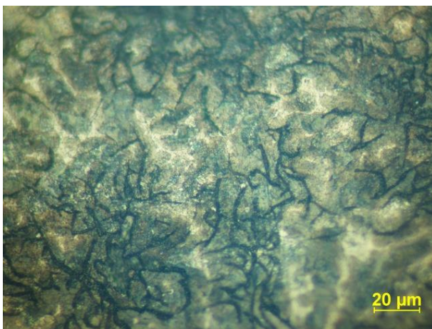
Obr. 3.18 Mikrostruktura pístního kroužku z litiny s lupínkovým grafitem – Nital, zvětšení 500násobné (10x50), kroužek č. 1
