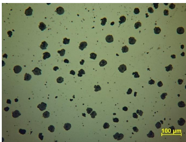
Obr. 3.28 Mikrostruktura pístního kroužku, litina s kuličkovým grafitem – neleptáno, zvětšení 100násobné, kroužek č. 3
