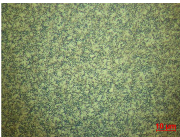
Obr. 3.24 Mikrostruktura pístního kroužku, ocel – Nitral, zvětšení 1000násobné (20x50), kroužek č. 2
