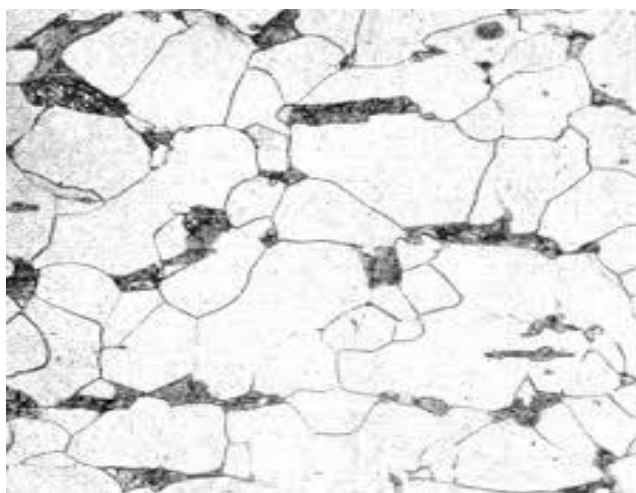
Obr. 2.14 Struktura chrom-křemíkové oceli pod mikroskopem
