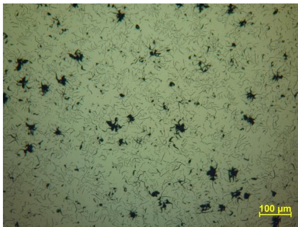
Obr. 3.15 Mikrostruktura pístního kroužku z litiny s lupínkovým grafitem – neleptáno, zvětšení 100násobné (8x12,5), kroužek č. 1
