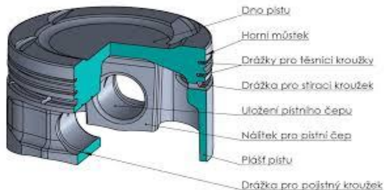
Obr. 2.2 Umístění pístních kroužků na pístu [7]
