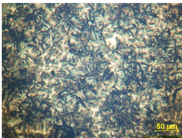
Obr. 3.17 Mikrostruktura pístního kroužku z litiny s lupínkovým grafitem – Nital, zvětšení 250násobné (20x12,5), kroužek č. 1
