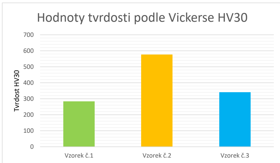
Obr. 3.32 Grafické zobrazení hodnot tvrdostí pístitních kroužků (č. 1, 2 a 3), zkouška tvrdosti podle Vickerse
