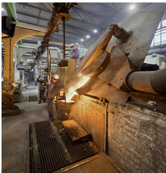
Obr. 3.6 Indukční středofrekvenční pec, vylévání taveniny litiny pro výrobu pístních kroužků do lící pánve
