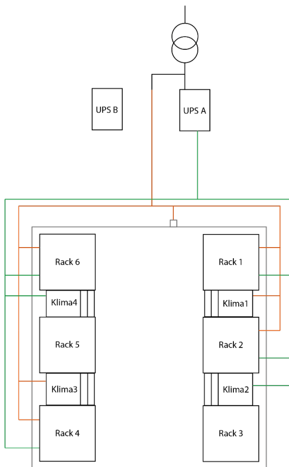
Obr 23 Zjednodušené schéma energetických rozvodů serverovny v High-tech technologickém-výukovém pavilonu Fakulty lesnické a dřevařské na České zemědělské univerzitě
