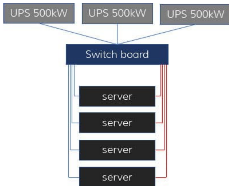
Obr 1 Schéma architektury N+1
