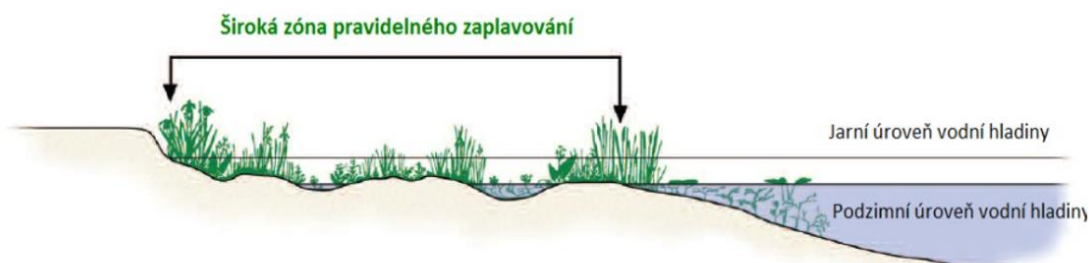
Obr. 15 Hloubení tůň – zásada členité a široké zóny pravidelného zaplavování [20]
