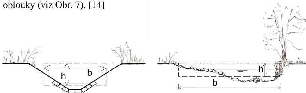
Obr. 6 Srovnání příčných profilů technického a přirozeného koryta [14]
