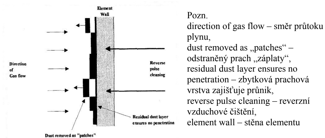
Obr. 3.6 Schematické znázornění čistícího mechanismu [11].
