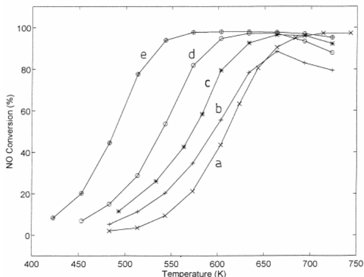
Obr. 3.1 Závislost NO konverze na teplotě: a) WO_3(9)/TiO_2 , b) V_2O_5(0,78)/TiO_2 , c) V_2O_5(1,4)/TiO_2 d) V_2O_5(0,78)/WO_3(9)/TiO_2 , e) V_2O_5(1,4)/WO_3(9)/TiO_2 [7].
