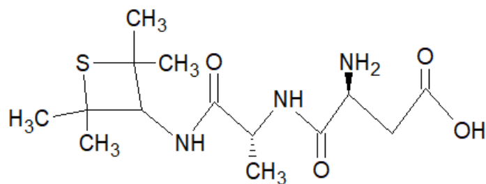
Obrázek 9 Strukturální vzorec Alitamu
