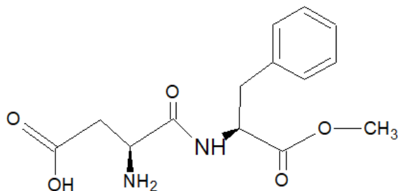
Obrázek 4 Strukturní vzorec Aspartamu
