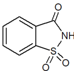
Obrázek 1 Strukturní vzorec Sacharinu
