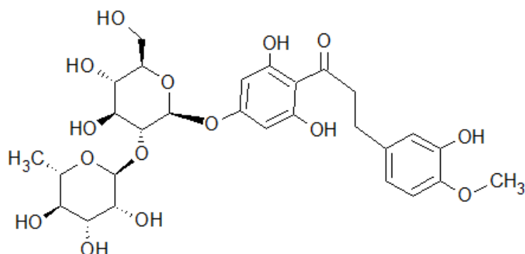
Obrázek 7 Strukturální vzorec Neohesperidinu dyhydrochalkonu
