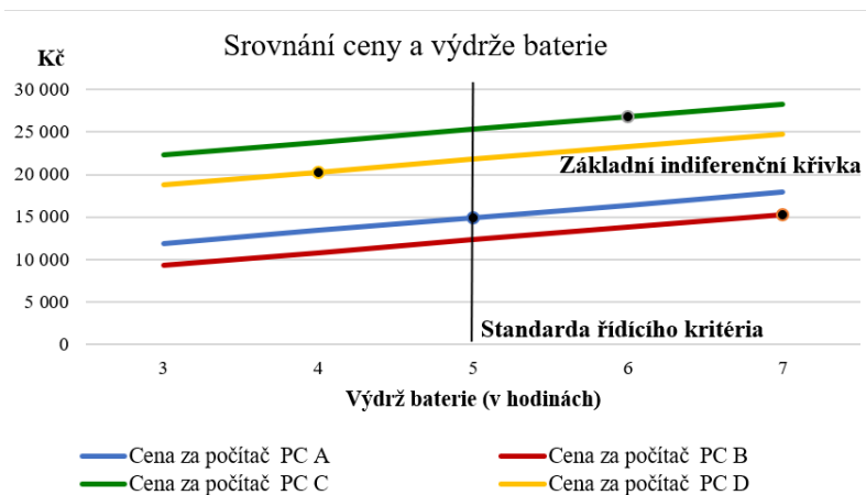
Graf č. 3 Ukázkový graf metody postupných substitucí (vlastní zpracování)
