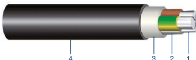
Obr. 5.3: Kabel AXEKCY [37]
