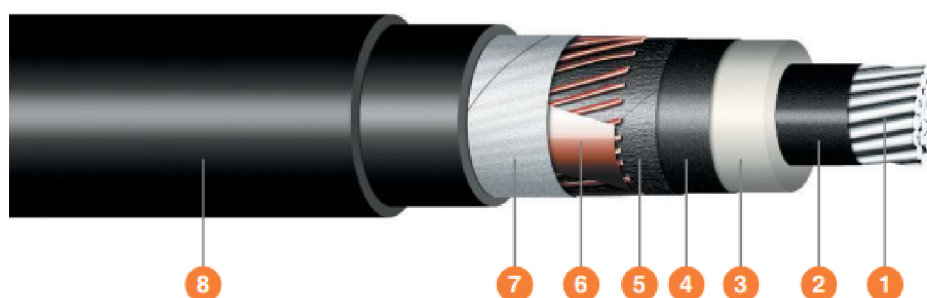
Obr. 5.1: Kabel AXEKVCEY [35]
