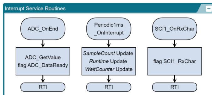
Obr. 21.: Vývojový diagram programu mikrokontroleru
