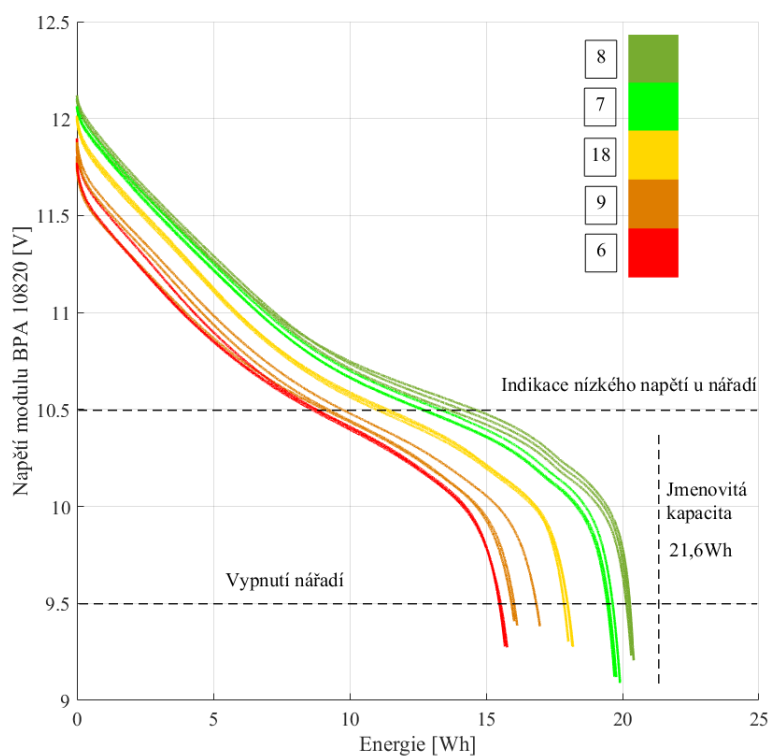
Obr. 26.: Průběh napětí při vybíjení modulu BPA 10820 v závislosti na energii
