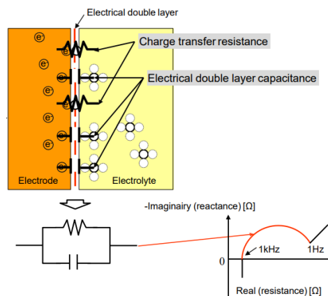
Obr. 10.: vliv přesunu náboje mezi elektrolytem a elektrodami [8].
