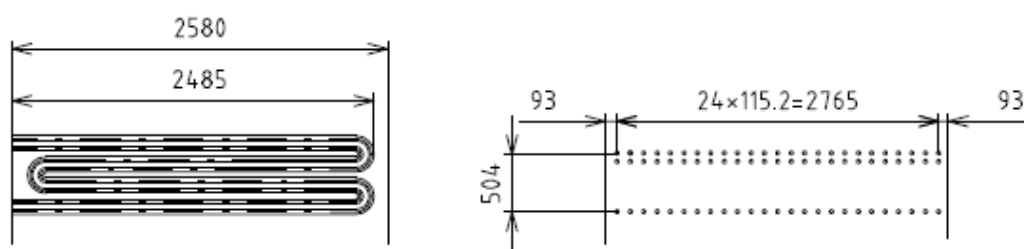
Obrázek 2 schéma přehříváku P2
