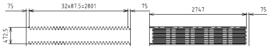
Obrázek 4 schéma přeříváku P1
