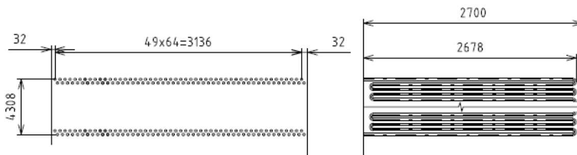
Obrázek 6 schéma ekonomizéru 1
