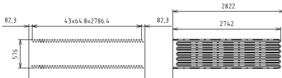
Obrázek 5 schéma ekonomizéru 2
