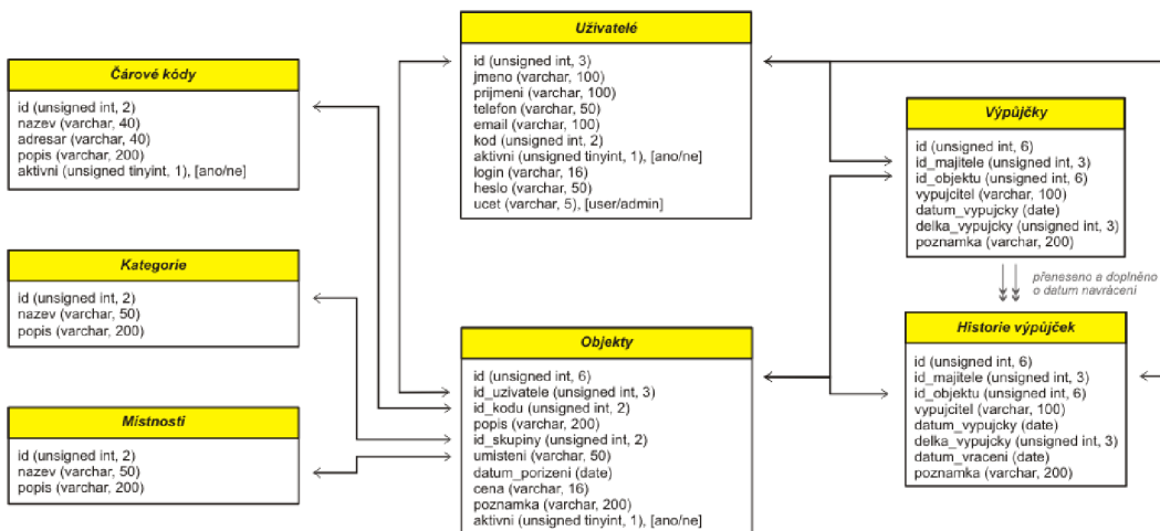
Obr. 7.2 Schéma MySQL databáze aplikace IS
