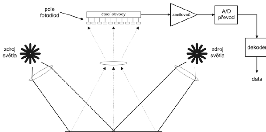
Obr. 6.3 Schéma CCD čtečky čárových kódů
