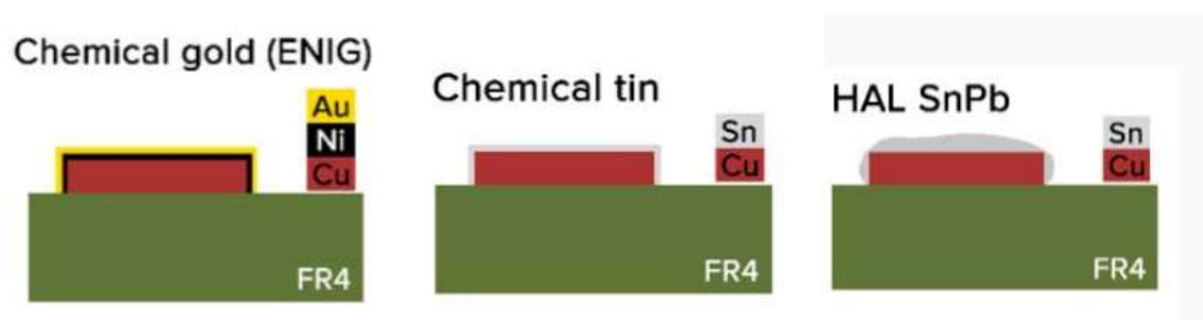
Obrázek 5.1 Struktura povrchových úprav, zprava imerzní zlato, imerzní cín a olovnatý HAL [14]
