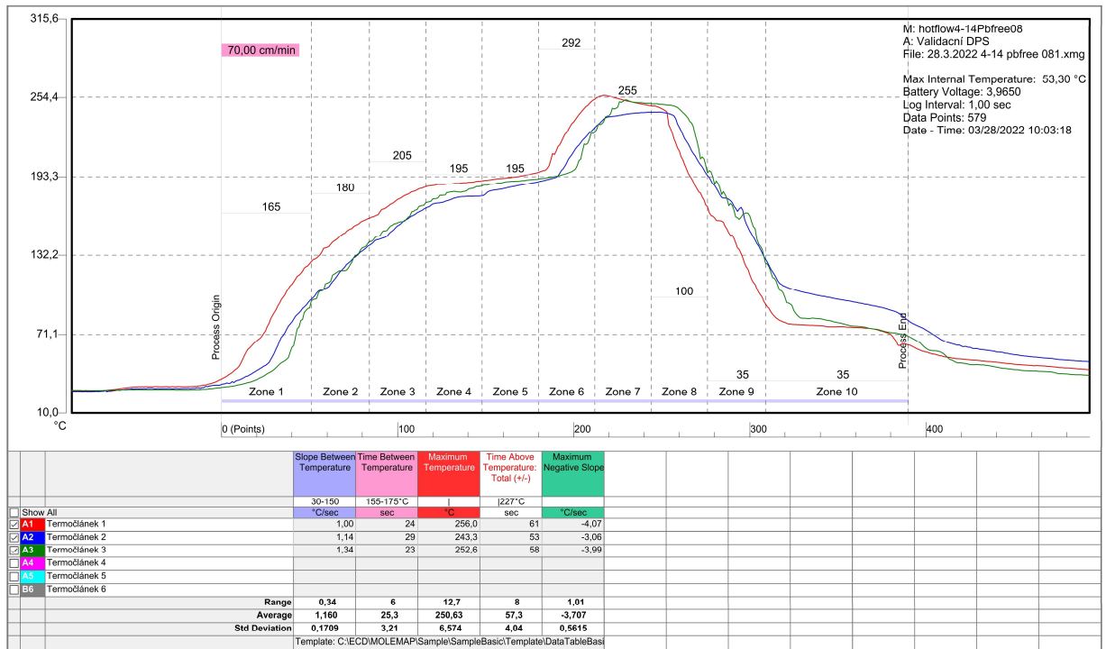
Obrázek 8.9 Teplotní profil TP2 měřený na peci Ersas 4/14
