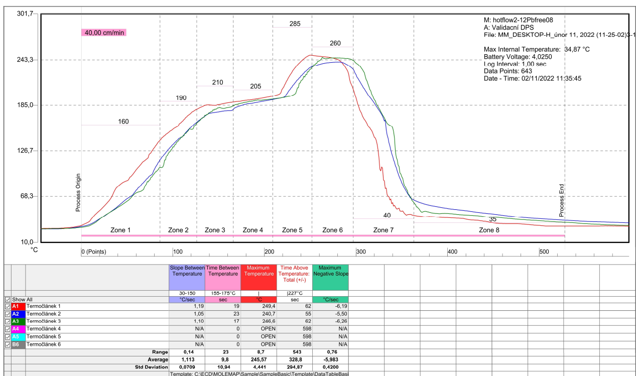
Obrázek 8.6 Teplotní profil TP2 měřený na peci Ersa 3/14
