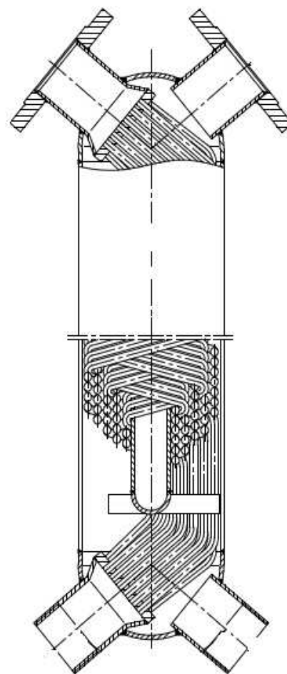
Obr. 6. Řez šroubovicového výměníku [9]
