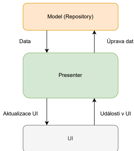
Obrázek 4.2: Model-View-Presenter
