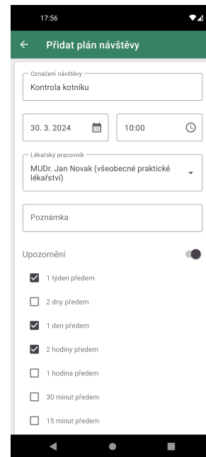
Obrázek 3.19: Nový plán
