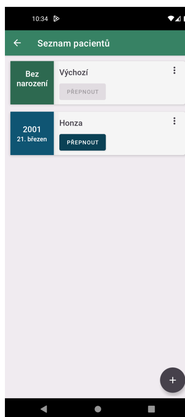
Obrázek 3.5: Výpis pacientů
