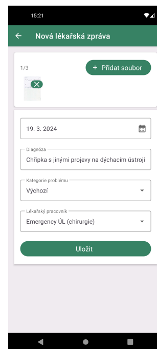
Obrázek 3.8: Nová zpráva
