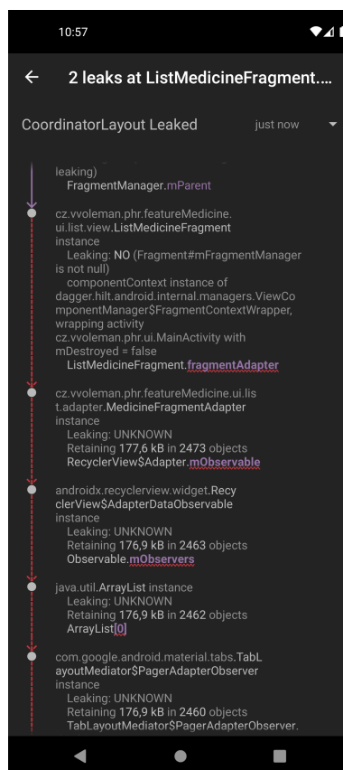
Obrázek 5.2: Stacktrace úniku
