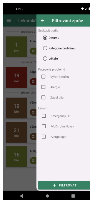
Obrázek 3.7: Filtrování
