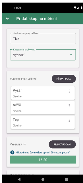
Obrázek 3.16: Nová skupina
