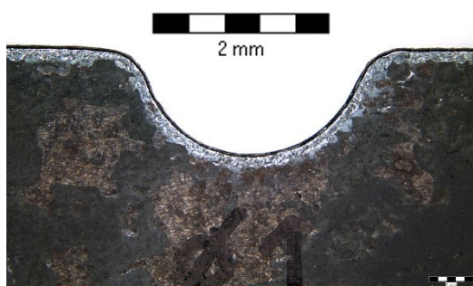
Obr. 46 Porovnání vzorků oceli S355, tl. 15 mm: A) Laser (vlevo), zvětšeno 6,3×. B) Vodní paprsek (vpravo), zvětšeno 6,3×.
