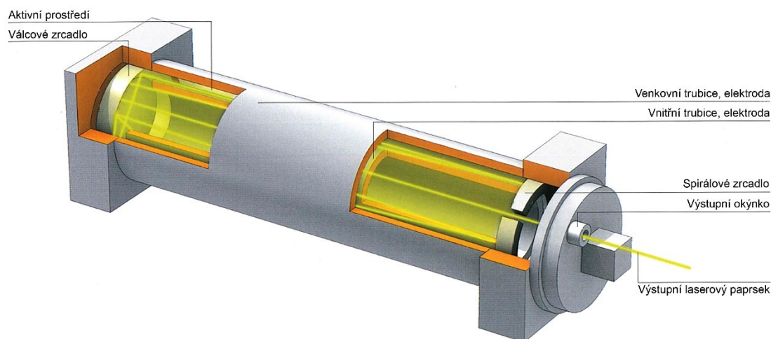
Obr. 13 Schéma Coax laseru [15].
