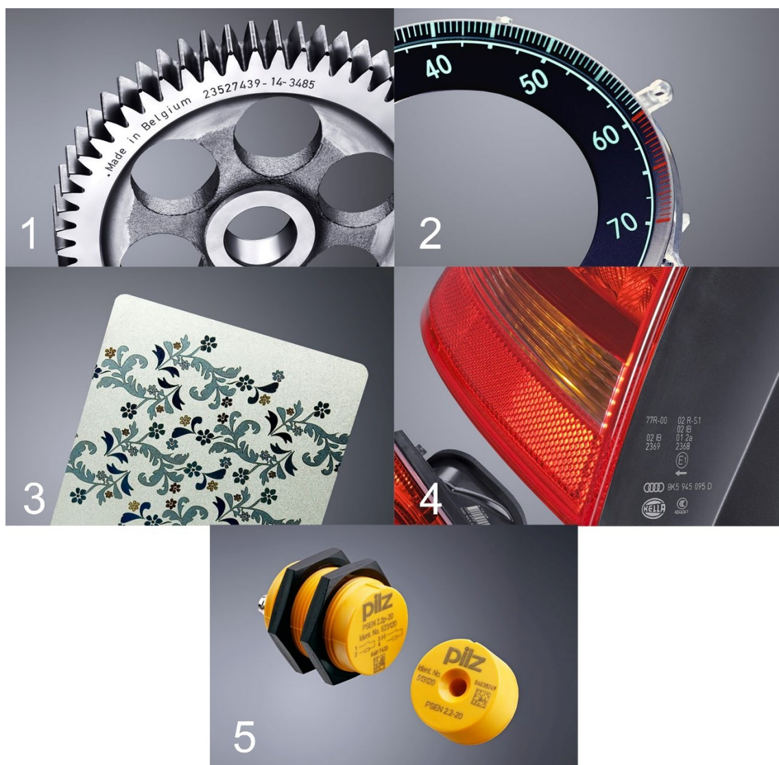
Obr. 25 Příkladů použití značení [15]: 1) gravírování 2) úběr 3) žíhání 4) zpěnění 5) zbarvení.
