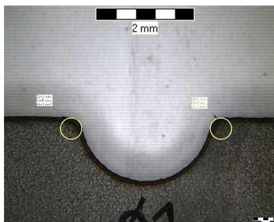
Obr. 40 Pohled na půlkruhové vybrání: A) Označené \varnothing 1 (vlevo), zvětšeno 6,3×. B) Měření zaoblení hran (vpravo), zvětšeno 6,3×.
