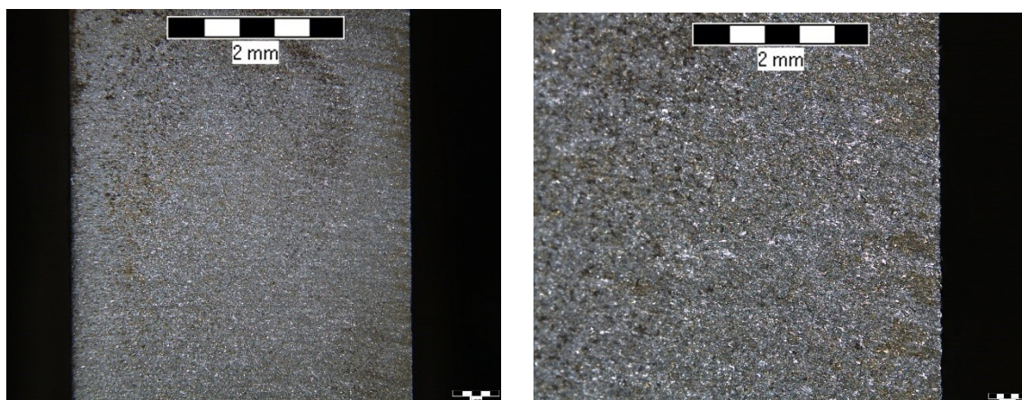
Obr. 52 Snímek plochy řezu oceli S355, vodní paprsek, tl. 15 mm: A) Zvětšení 6,3×. B) Zvětšení 20×.
