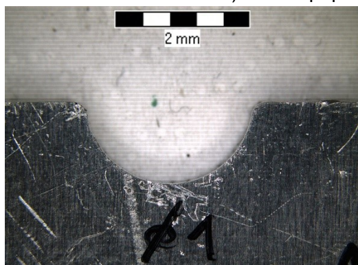
Obr. 44 Porovnání vzorků hliníkové slitiny EN AW 1050A H24, tl. 3 mm: A) Laser (vlevo), zvětšeno 6,3×. B) Vodní paprsek (vpravo), zvětšeno 6,3×.
