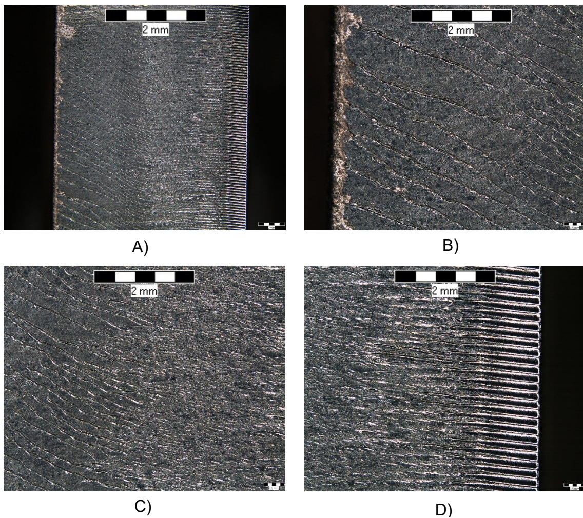
Obr. 51 Přehledový snímek ploch řezu oceli S355, laser, tl. 15mm: A) Celá plocha, zvětšení 6,3×, B) konec řezu, zvětšení 20×, C) Střední oblast, zvětšení 20×, D) Začátek řezu, zvětšení 20×.
