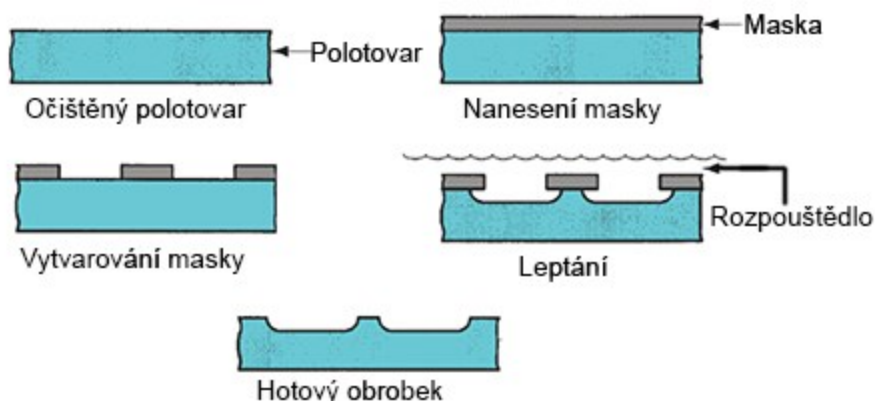
Obr. 4 Jednotlivé kroky chemického obrábění [8].
