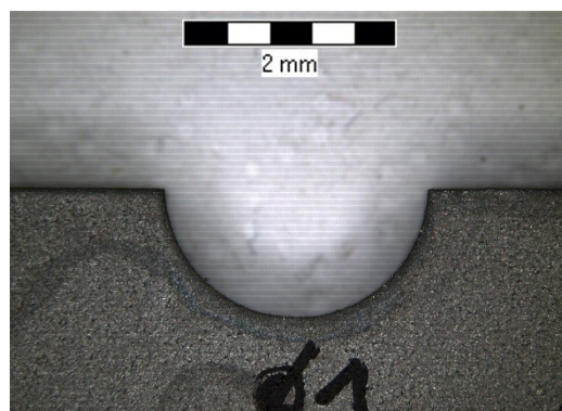
Obr. 43 Porovnání vzorků AISI 304L, tl. 5 mm: A) Laser (vlevo), zvětšeno 6,3×. B) Vodní paprsek (vpravo), zvětšeno 6,3×.
