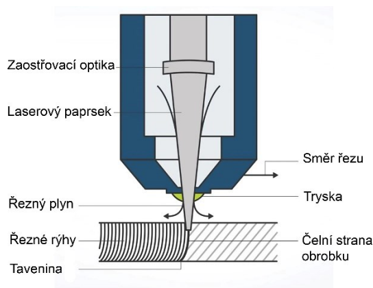
Obr. 20 Proces řezání [26].
