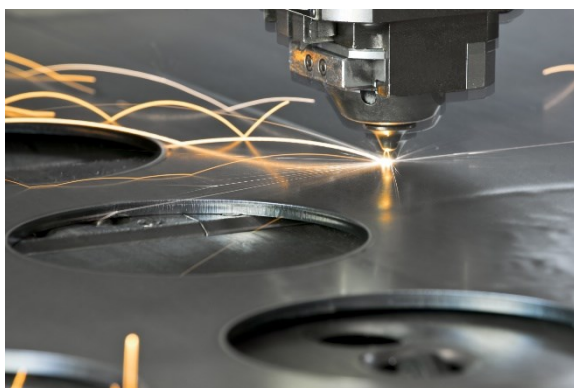
Obr. 19 Řezání laserem [15].
