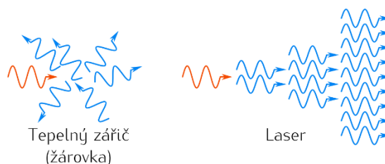
Obr. 9 Srovnání emise záření běžného zdroje a laseru [16].
