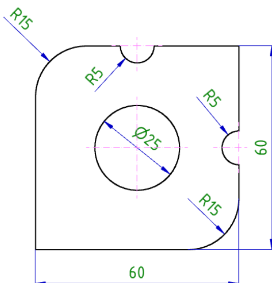
Obr. 37 Model vzorku s rozměry.
