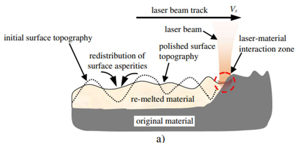
Obr. 3-6 Schéma laserového leštění [35]
