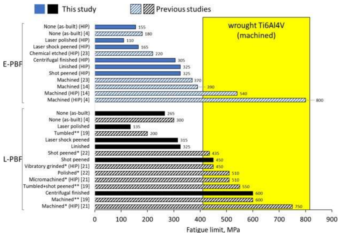
Obr. 4-1 Porovnání metod na únavovou životnost vzorků [38]
