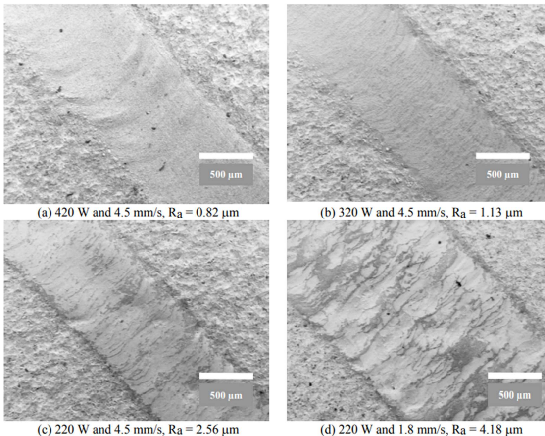
Obr. 3-7 Povrch po laserovém leštění v závislosti na parametrech [33]
