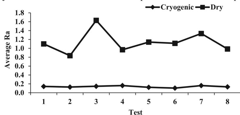
Obr. 3-2 Výsledná drsnost povrchu obrábění při kryogenní teplotě [13]
