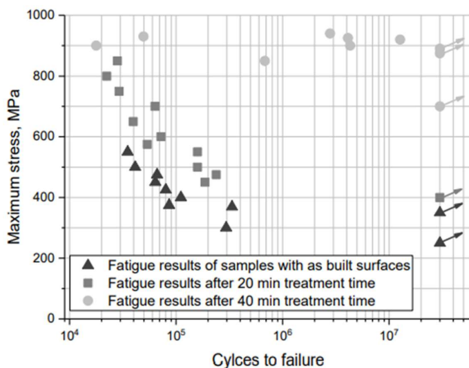
Obr. 3-11 Únavová životnost elektrolyticky leštěných vzorků [51]
