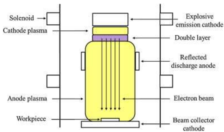
Obr. 3-8 Schéma pro metody využívající elektronový paprsek [44]
