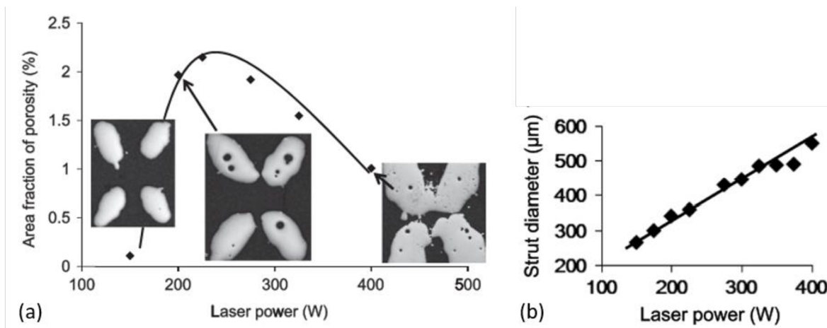
obr. 2-4 (a) Graf závislost porozity na výkonu laseru při konstantní skenovací rychlosti doplněný o snímky z mikroskopu; (b) graf závislosti průměru prutu na výkonu laseru. [6]
