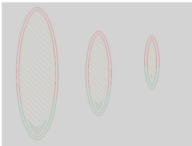
obr. 4-4 Použité skenovací strategie pro všechny průměry vyráběné pod úhlem 20°. Zeleně jsou upravené oblasti převisů, červeně obrysy a žlutě jsou výplně.
