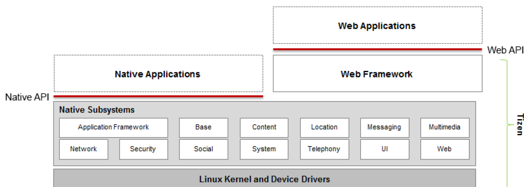
Obrázek 5.2: Hierarchie platformy Tizen (viz sekce Tizen Application Types v dokumentaci [48])
