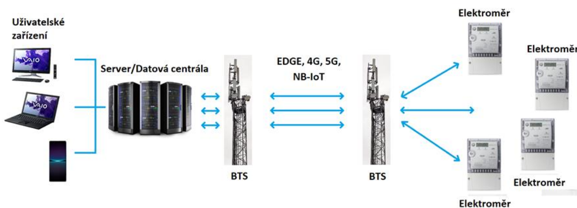
Obr. 8 komunikace elektroměrů bod vs. bod
