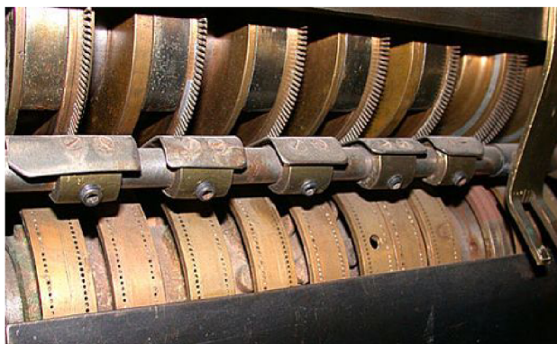
Obrázek 2.6: Válec pro rotační perforaci, převzato z [?]
