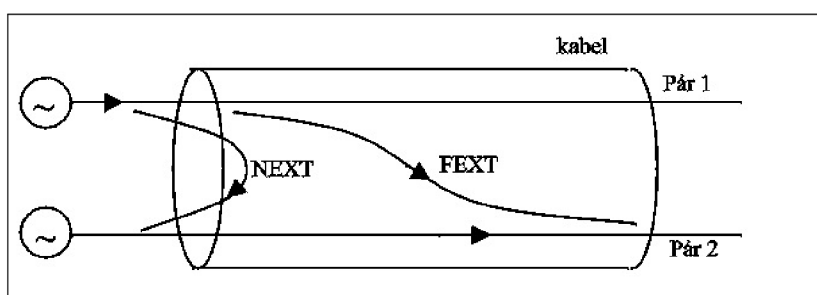
Obr. 2.1: Přeslechy [8]
