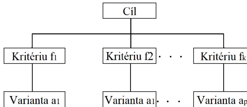
Obrázek 1 – Hierarchická struktura
