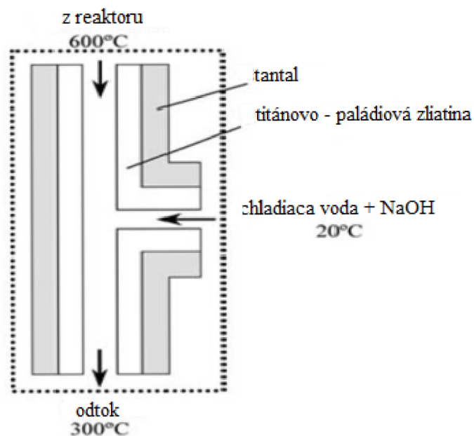
Obrázok č. 5: Kompozícia SCWO reaktoru pre zachádzanie s PCB (a) a pohľad z rezu zmiešavacej tuby (b).
