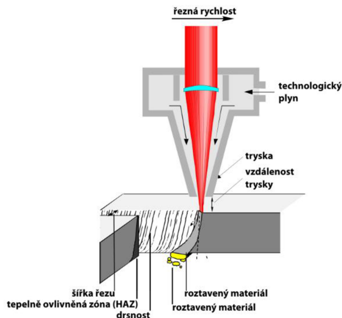
Obr. 2 Princip laserového řezání [5].
