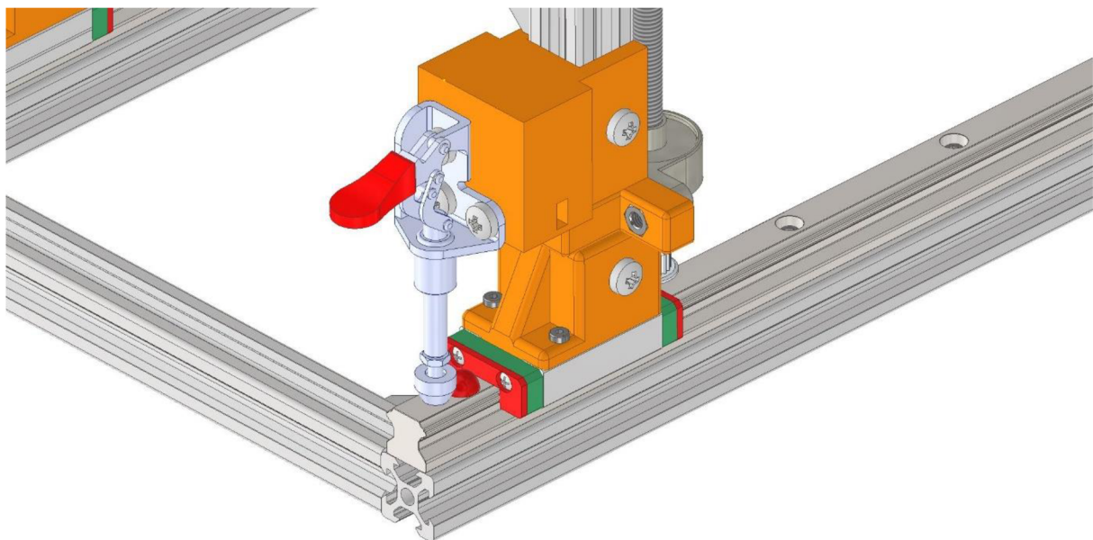
Obr. 20 Připevňená vertikální svorka k profilu.
