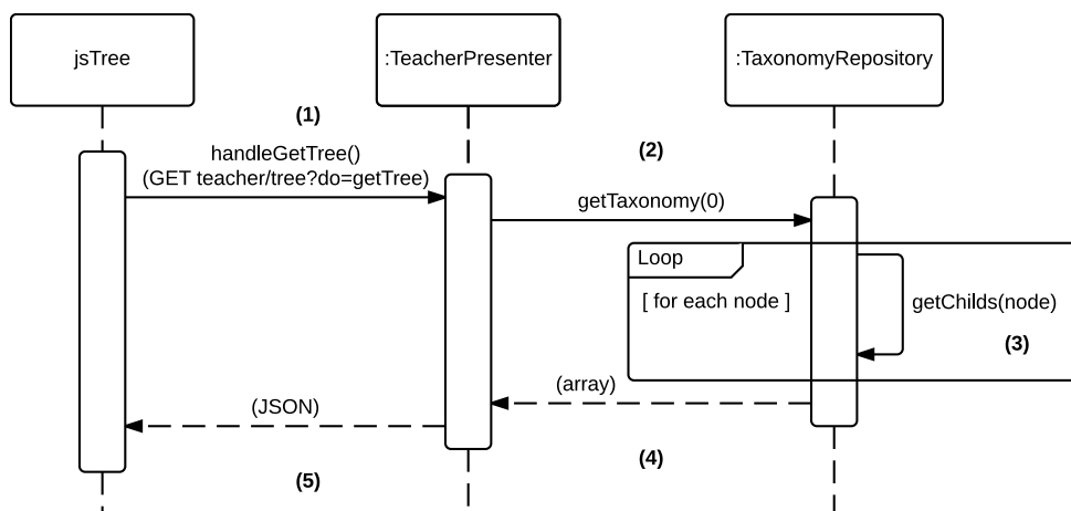
Obrázek 6.2: Sekvenční diagram zobrazení taxonomického stromu
