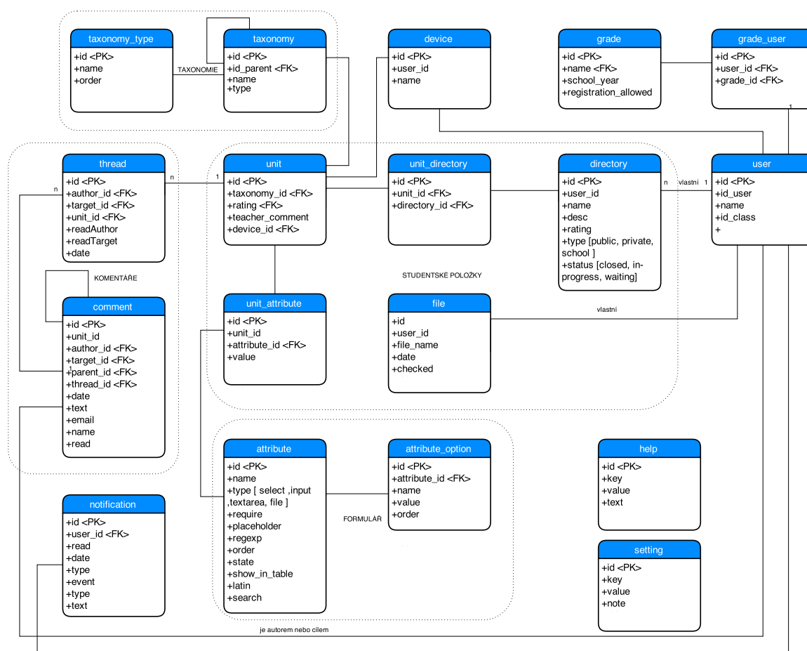
Obrázek C.1: Databázové schéma
