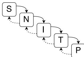
Obrázek 3.1: Vodopádový model
