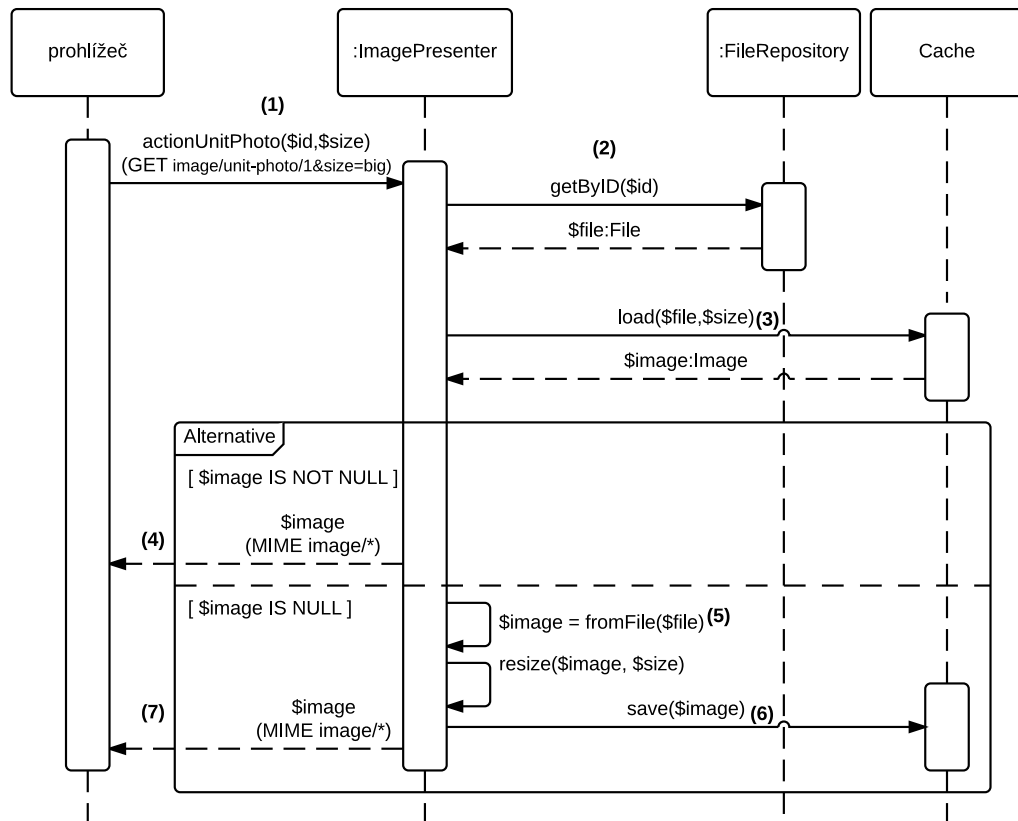
Obrázek 6.3: Sekvenční diagram získání obrázků
