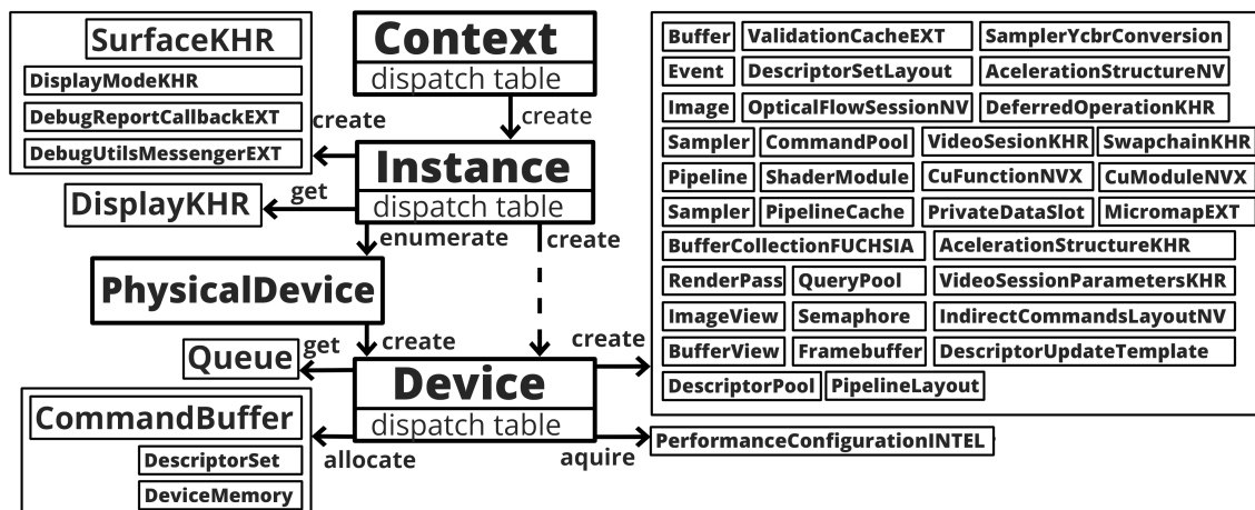
Obr. 3.2: Hierarchia objektov v novom RAII rozhraní
