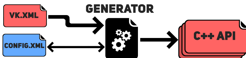
Obr. 3.3: Schéma generátora
