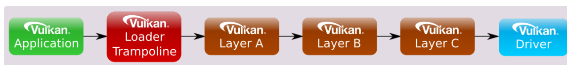
Obr. 2.3: Retazec volaní úrovně Device. Prevzaté z [18].
