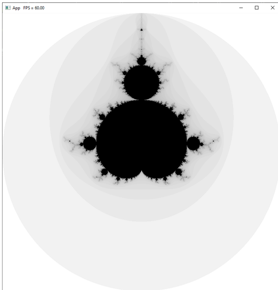
Obr. 6.3: Ukážková aplikácia
