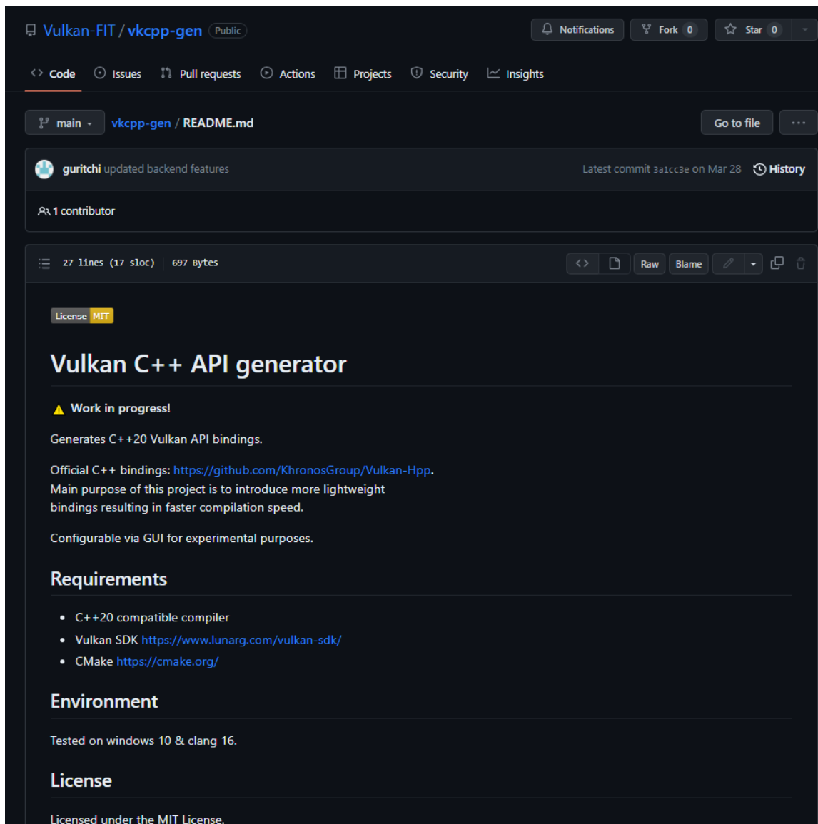
Obr. 6.4: Repoziár projektu
