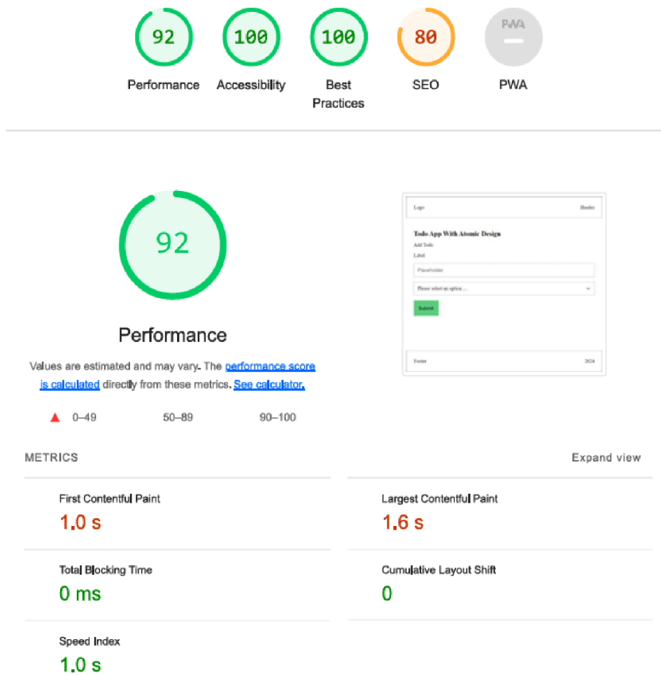
Obrázek č. 22 Výsledky Performance Testu v.1, 29.2.2024
