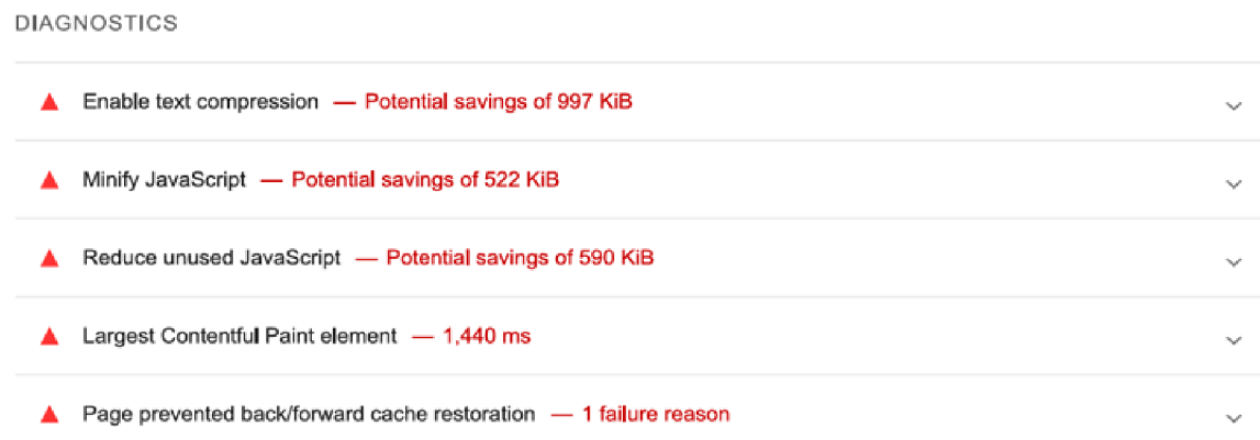
Obrázek č. 29 Výsledek bez atom. designu, 6.3.2024
