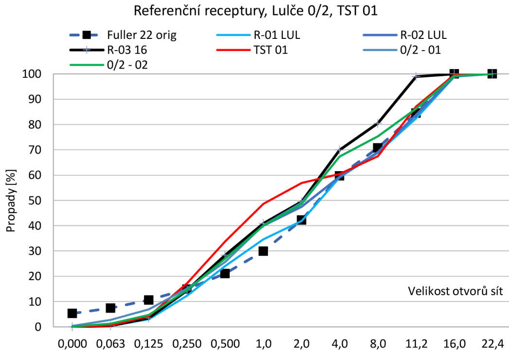
Obrázek 28: graf čar zrnitostí
