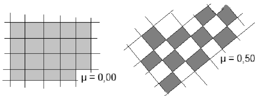
Obrázek 2: mezerovitost krychlí
