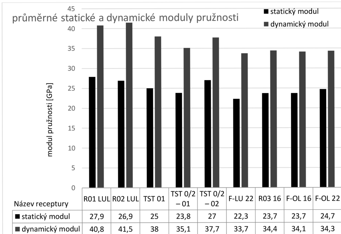
Obrázek 34: graf statických a dynamických modulů všech receptur s tabulkou hodnot
