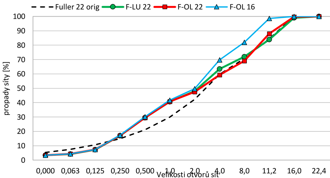
Obrázek 309: graf čar zrnitostí
