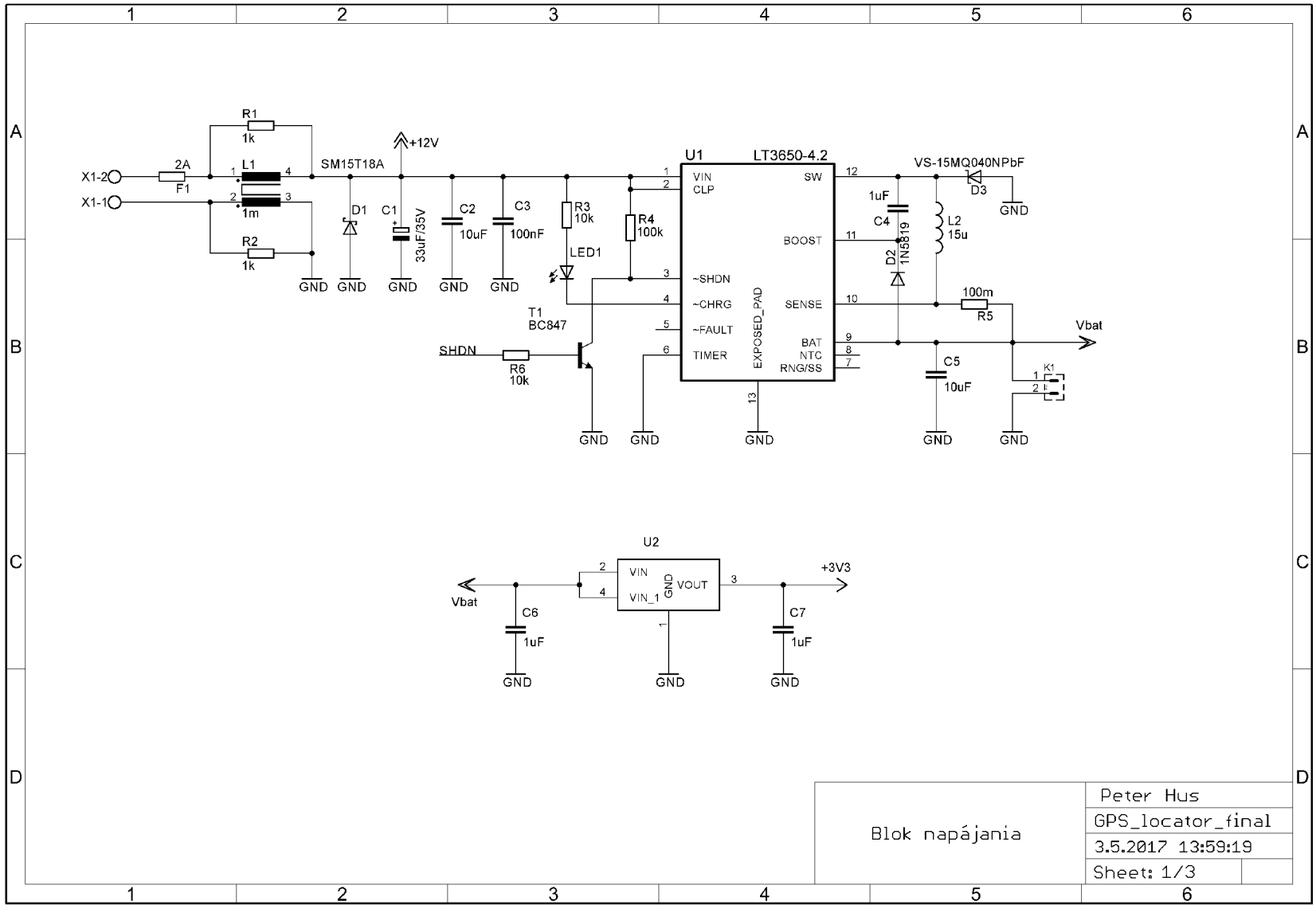
Schéma zapojenia napájacieho bloku
