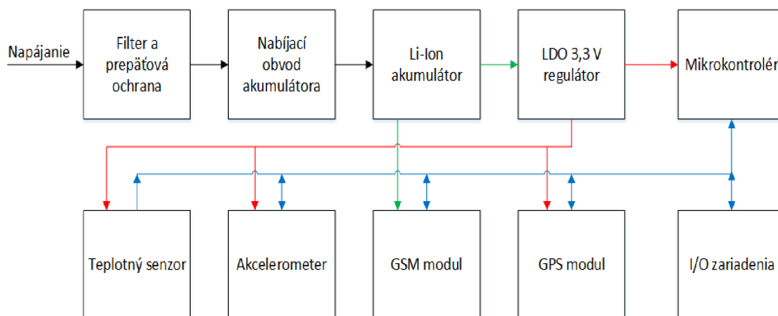
Obr. 3.1 Bloková schéma navrhovaného nízkopríkonového GPS prijímača
