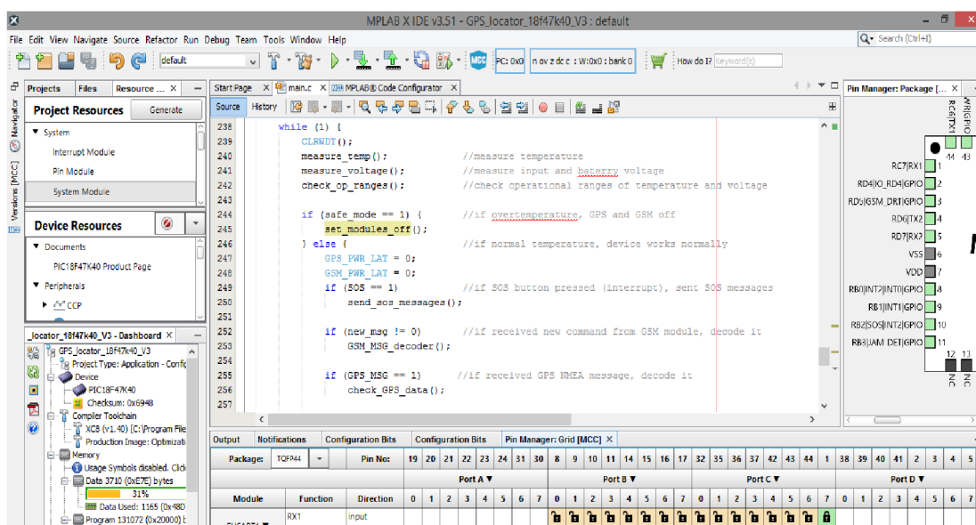
Obr. 6.1 Používateľské rozhranie programu MPLAB X
