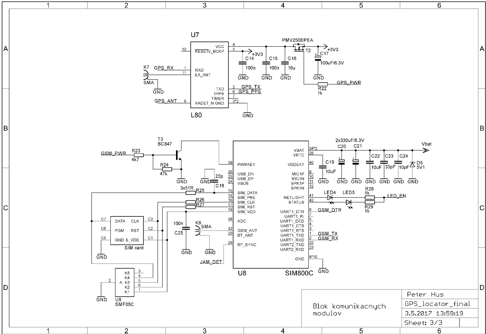
Schéma zapojenia bloku komunikačných modulov
