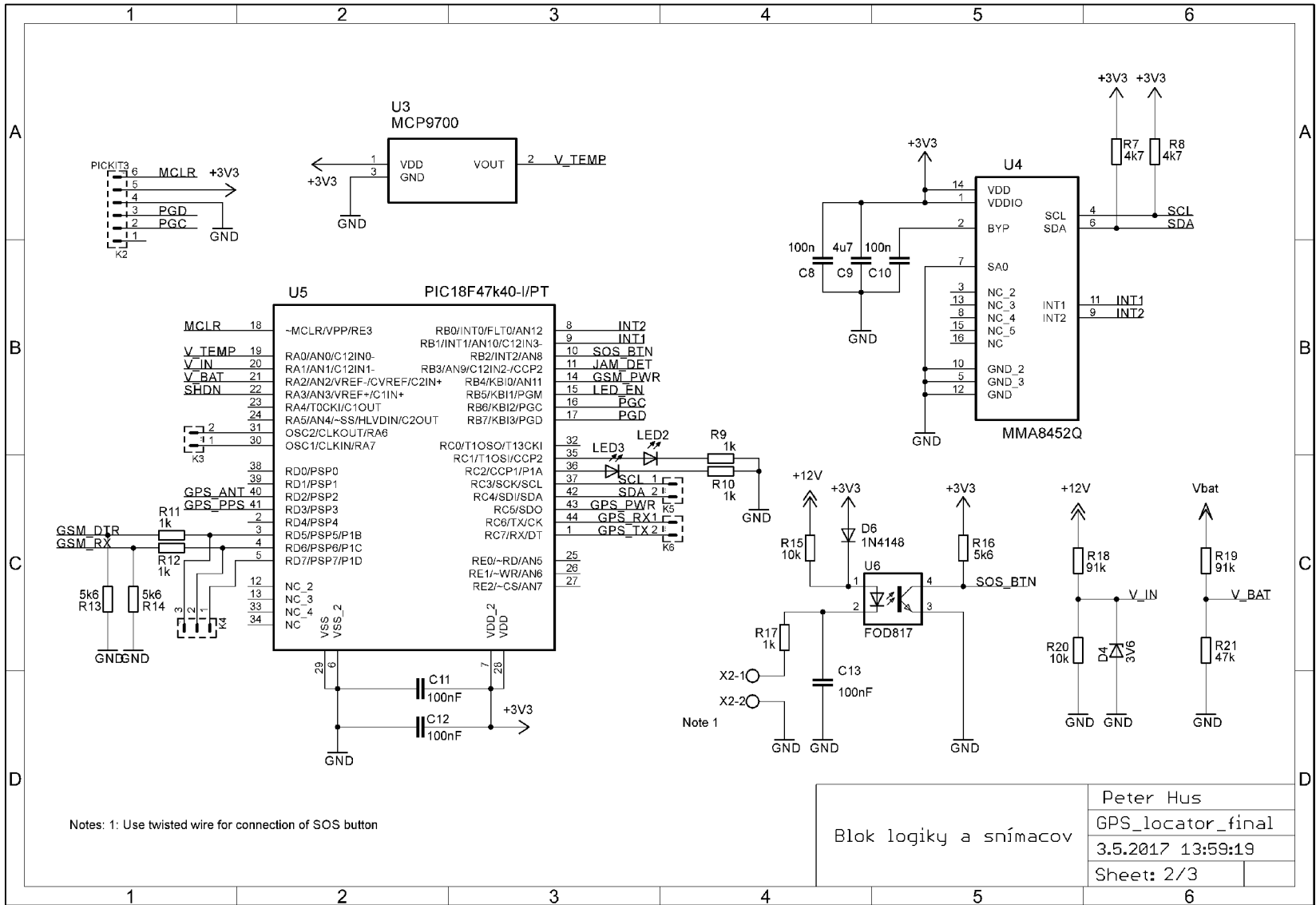
Schéma zapojenia bloku logiky a snímačov
