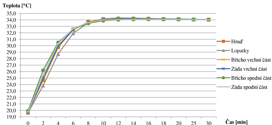
Obrázek 50: Graf zobrazující závislost povrchové teploty v závislosti na čase pro kontrolovanou oblast středu těla manekýna – náhřev č. 3
