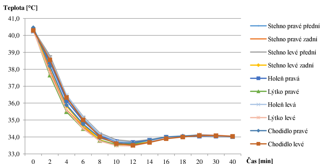
Obrázek 67: Graf zobrazující závislost povrchové teploty v závislosti na čase pro kontrolovanou oblast dolních končetin manekýna – chladnutí
