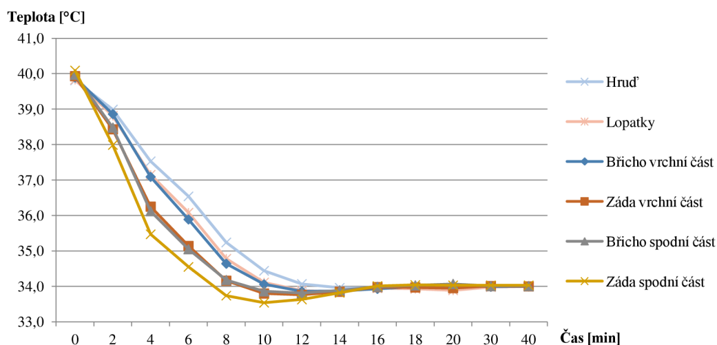
Obrázek 65: Graf zobrazující závislost povrchové teploty v závislosti na čase pro kontrolovanou oblast středu těla manekýna – chlazení
