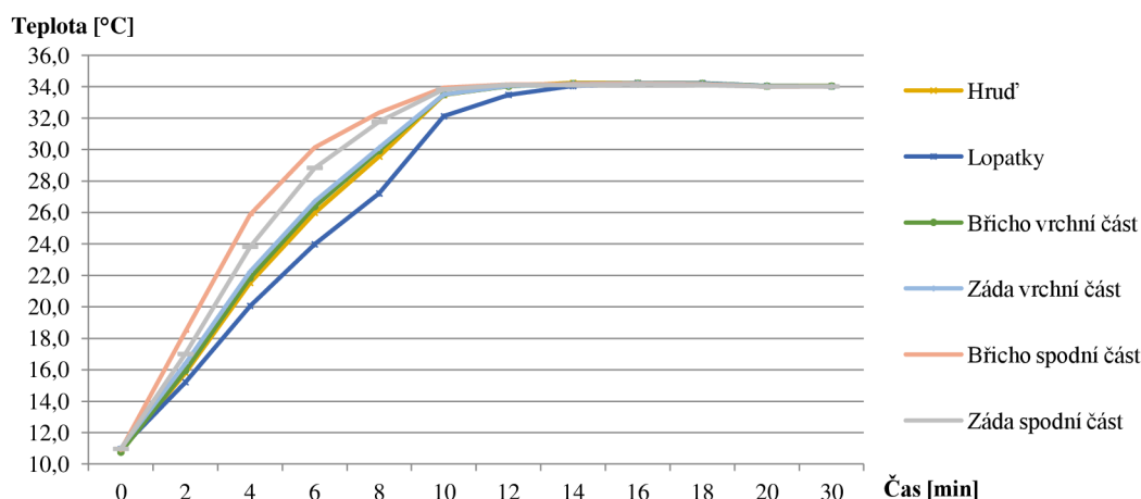
Obrázek 55: Graf zobrazující závislost povrchové teploty v závislosti na čase pro kontrolovanou oblast středu těla manekýna – náhřev č. 4
