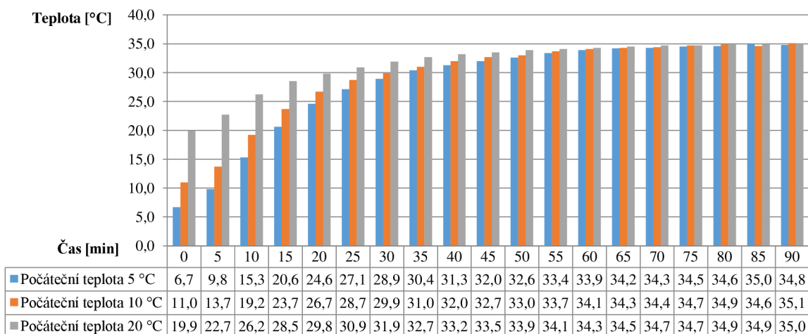
Obrázek 33: Graf náhřevu z počátečních teplot 5 °C, 10 °C, 20 °C a ustálení jejich hodnot pro termočlánek umístěný v hrudníku manekýna.
