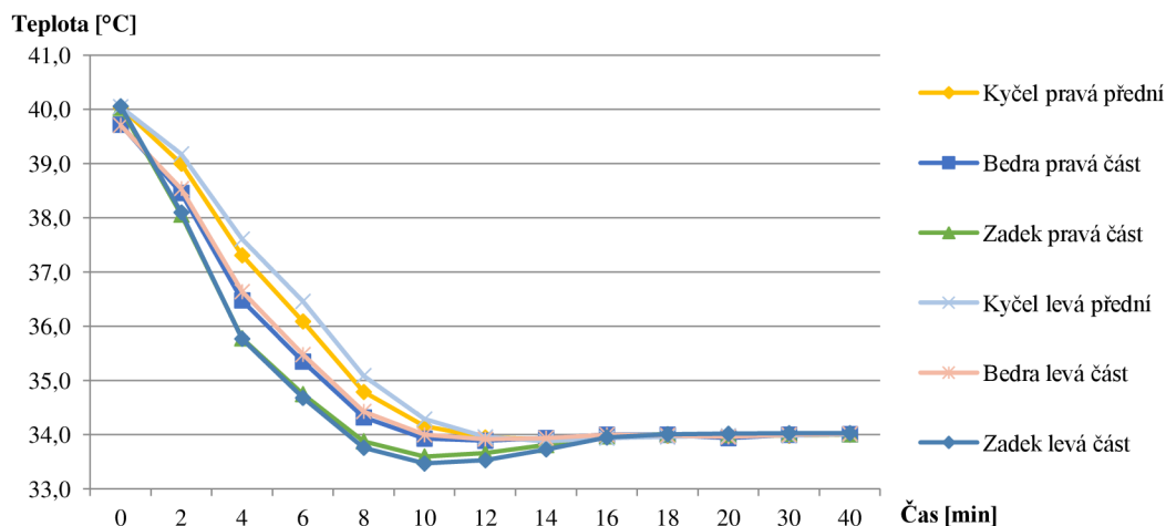
Obrázek 66: Graf zobrazující závislost povrchové teploty v závislosti na čase pro kontrolovanou oblast bederní části manekýna – chlazení
