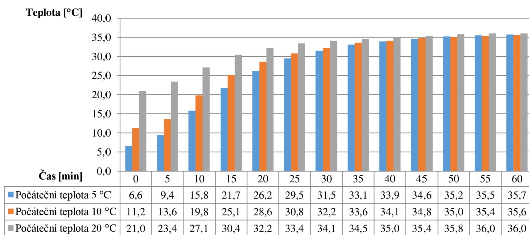
Obrázek 34: Graf náhřevu z počátečních teplot 5 °C, 10 °C, 20 °C a ustálení jejich hodnot pro termočlánek umístěný v předloktí manekýna.
