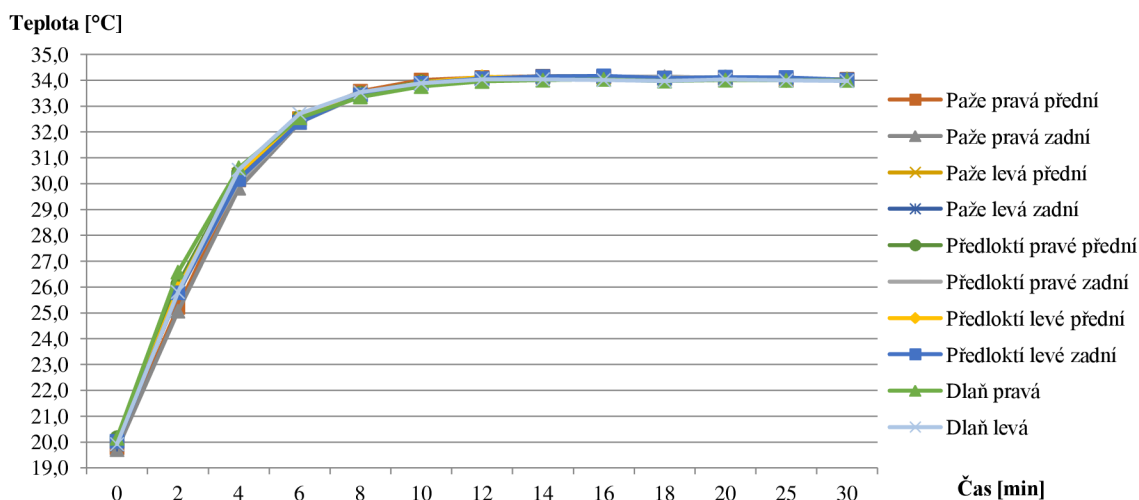
Obrázek 49: Graf zobrazující závislost povrchové teploty v závislosti na čase pro kontrolovanou oblast horních končetin manekýna – náhřev č. 3
