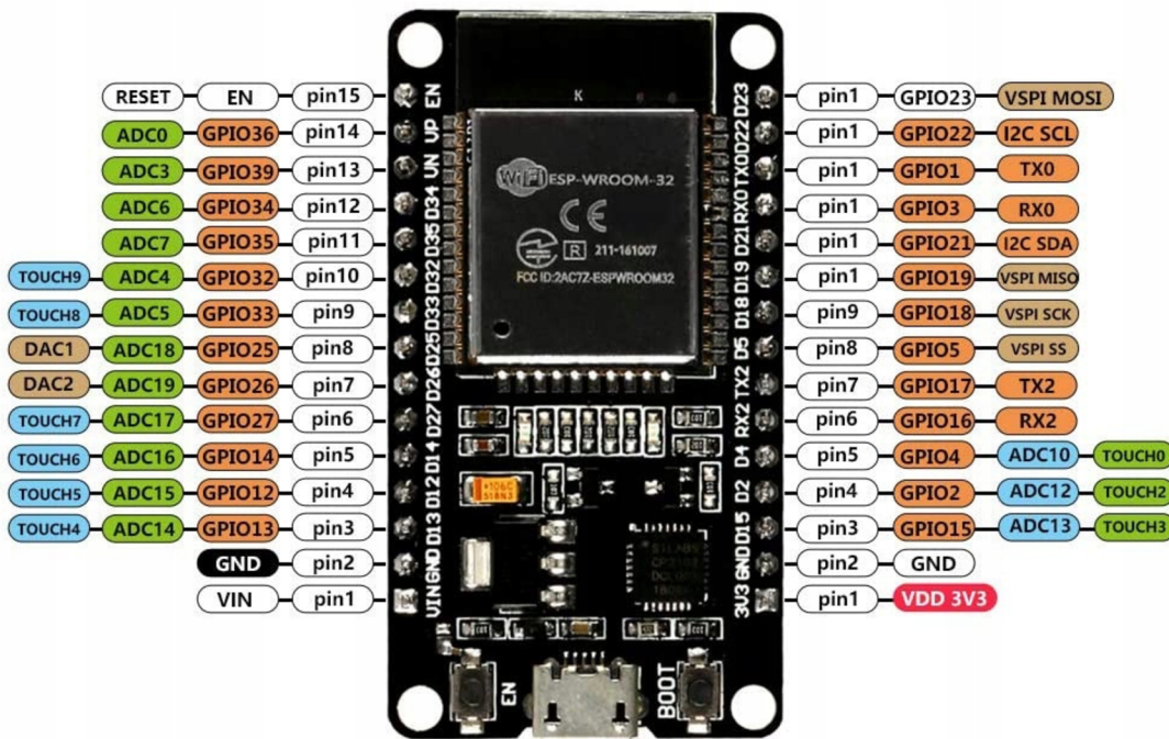
Obrázek 13 ESP32 a popis jednotlivých pinů
