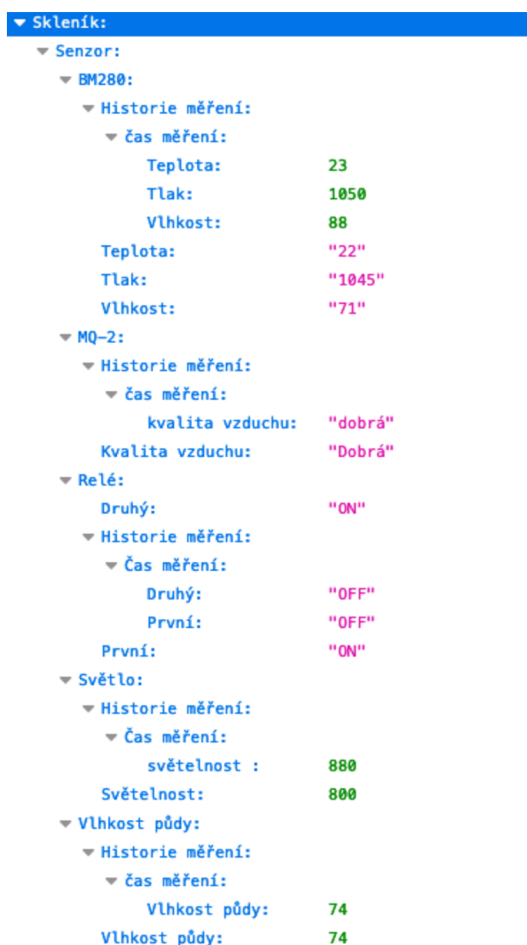
Obrázek 15 Struktura databáze
