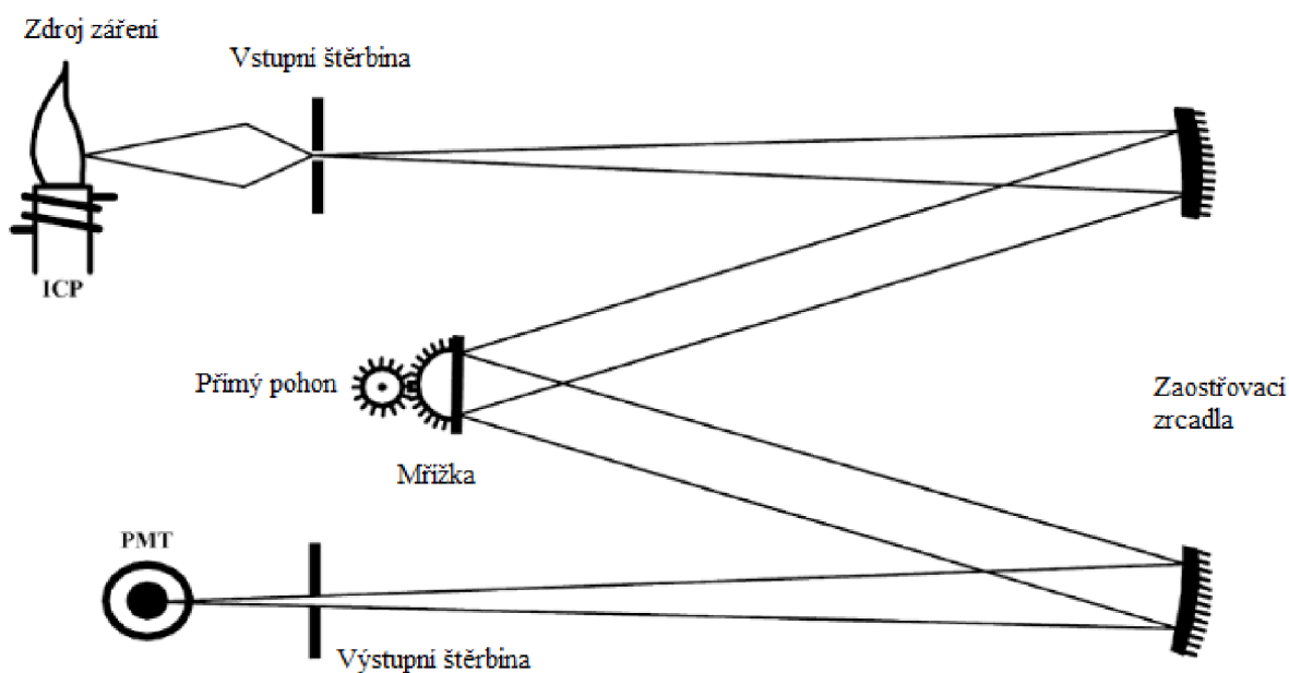
Obrázek 4: Czerny-Turner monochromátor (3)
