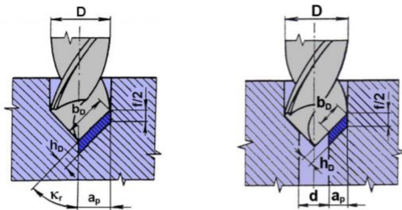
Obrázek 2.9. Průřez třísky [12].
