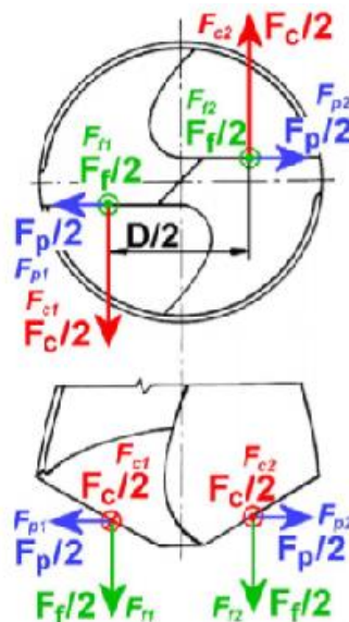
Obrázek 2.10. Složky řezných sil při vrtání [12].
