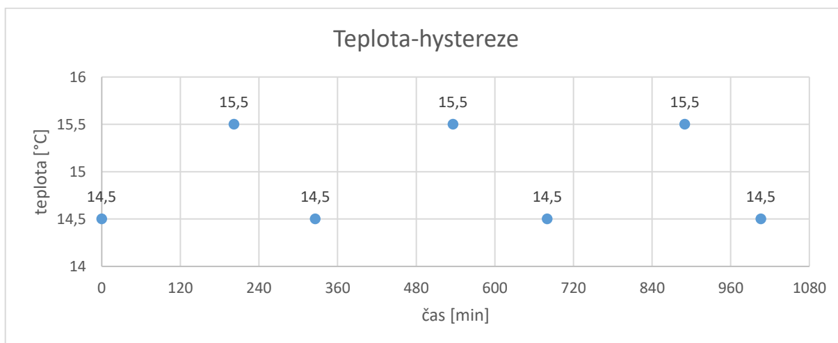
Obr. 12) Ověření funkce - teplota
