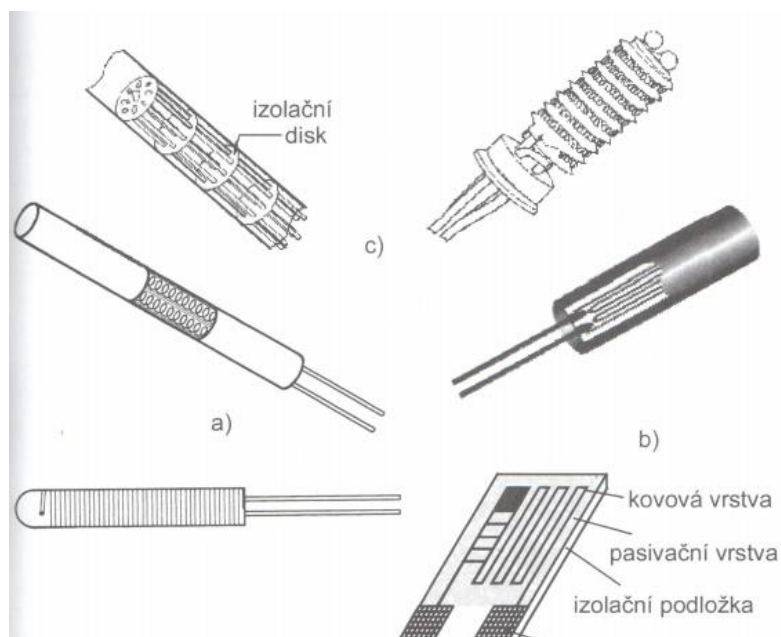
Obr. 2) Konstrukce měřicích odporů. [1]
