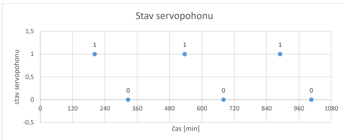
Obr. 13) Ověření funkce – stav servopohonu
