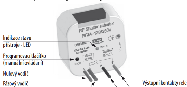
Obrázek 2.10 Jednotka RFJA [14].
