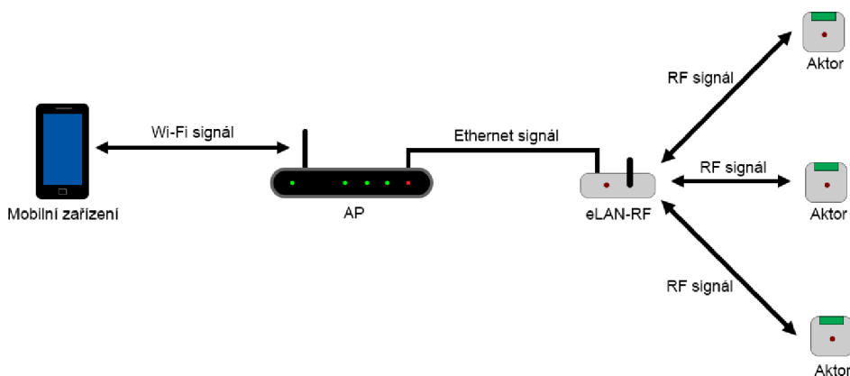
Obrázek 3.2 Schéma komunikace.
