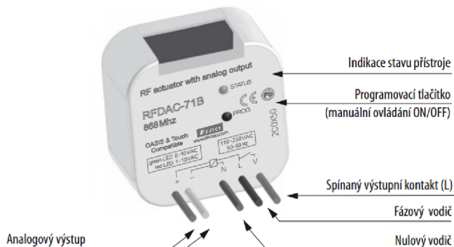
Obrázek 2.12 Jednotka RFDAC-71B [14].
