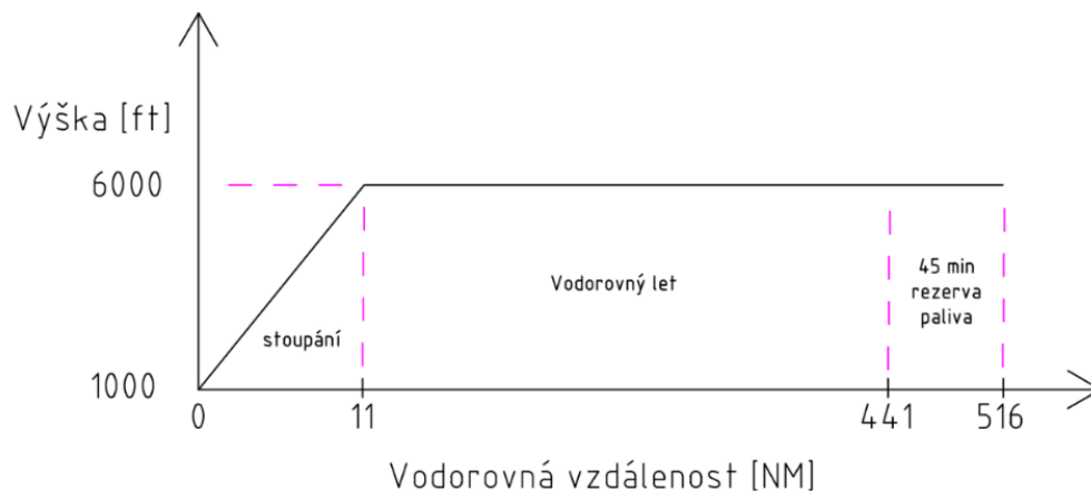
Obr. 2 Profil letu
