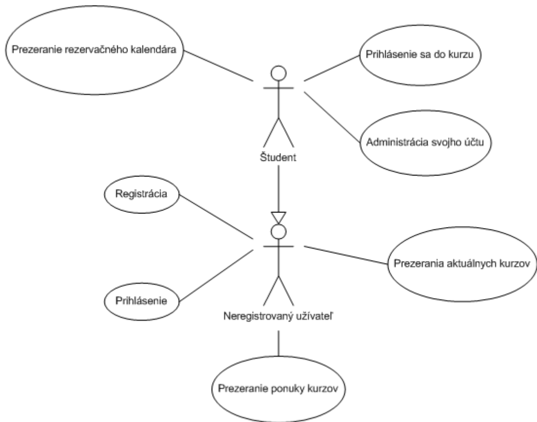
Obr. 3.2: Diagram prípadov použitia – Študent a neregistrovaný užívateľ
