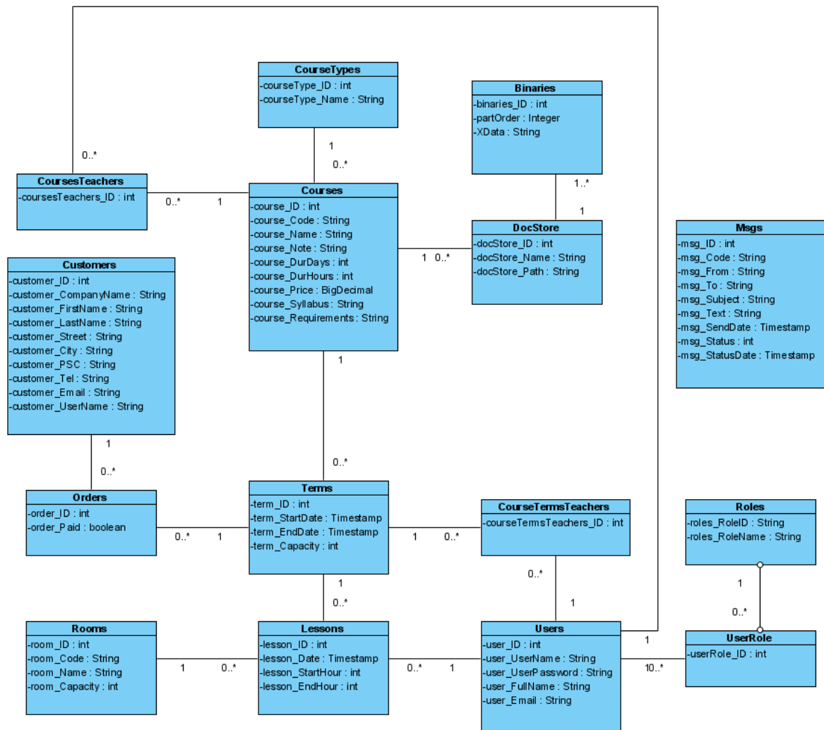
Obr. 3.3 ER diagram
