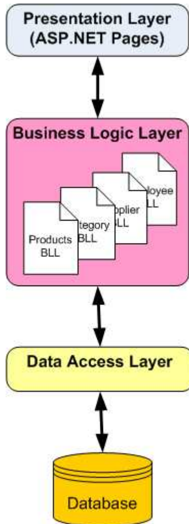
Obr. 3.5.1: Viacvrstvá architektúra aplikácie [7]
