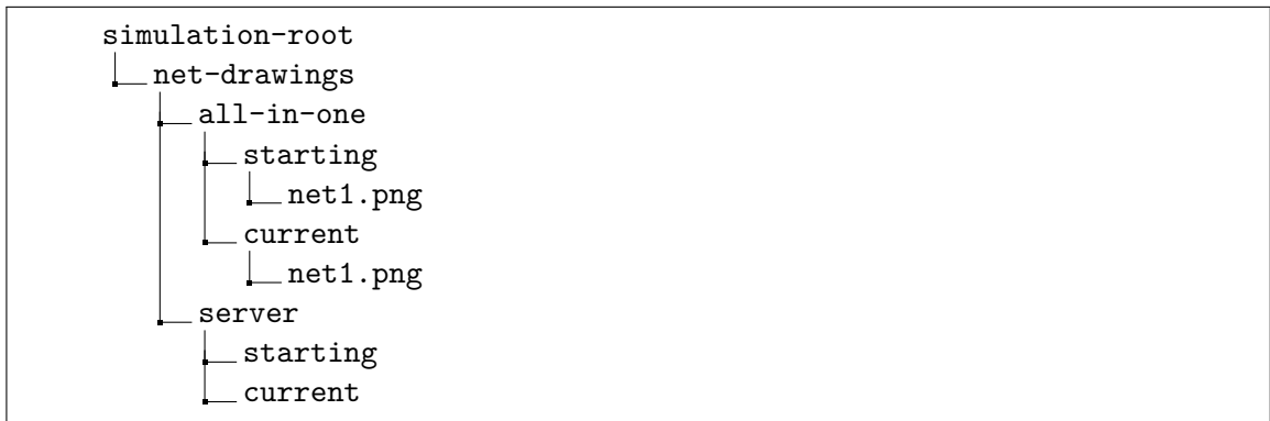
Obrázek 4.9: Struktura uložení zobrazení Petriho sítí.
