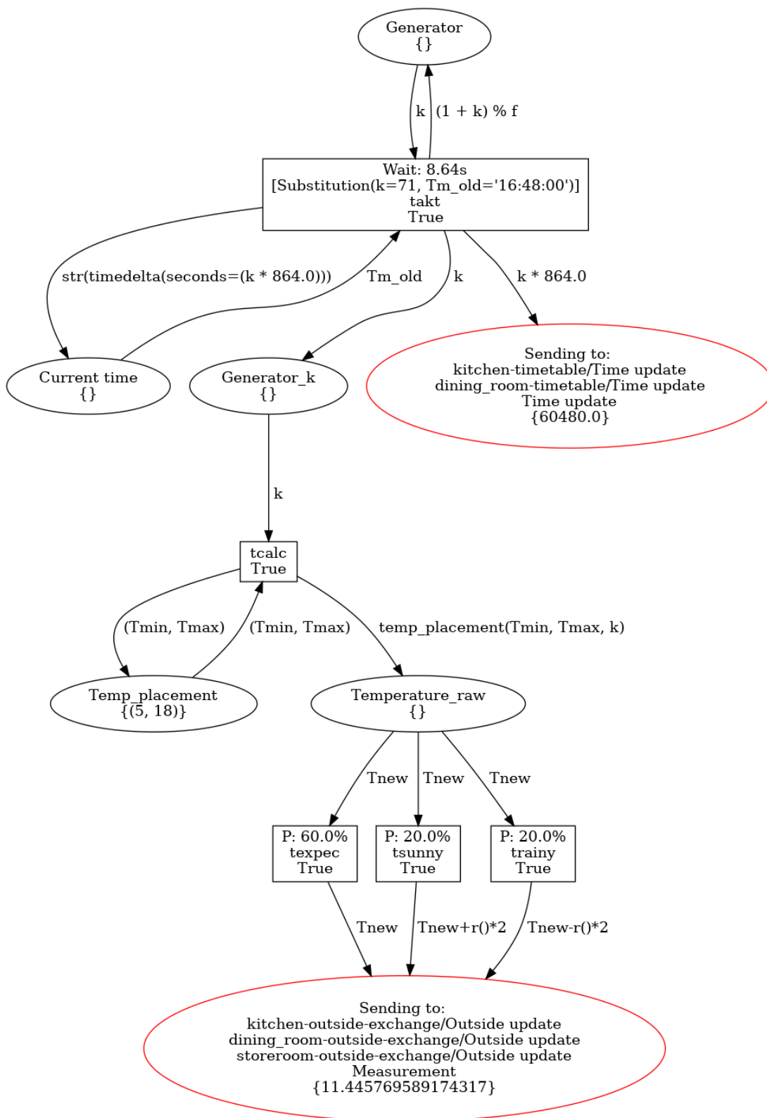
Obrázek 6.1: Simulace počasí a času.
