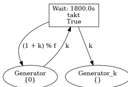
Obrázek 7.1: Generator doby dne.
