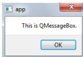
Obrázok 3.2: QMessageBox
