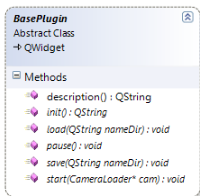
Obrázok 5.4: Trieda BasePlugin
