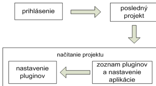
Obrázok 4.7: Načítanie aplikácie
