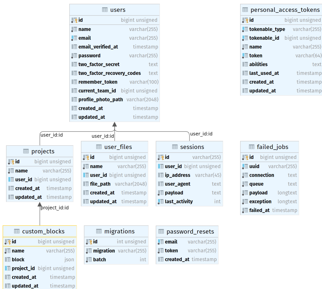
Obrázek 5.2: Schéma databáze
