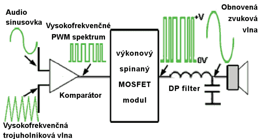
Obrázok 1.3 Popis fungovania triedy D [2]
