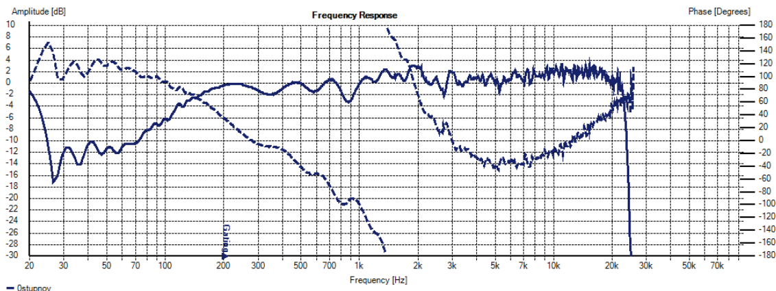
Obrázok 3.14 Meranie reprobredne signálom Square Noise, uhol 0°
