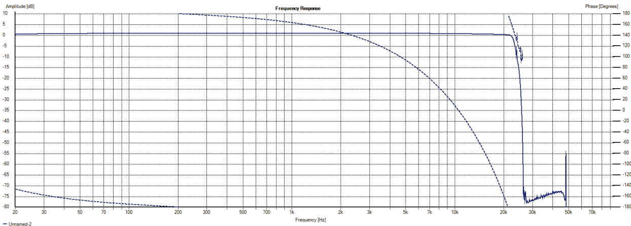
Obrázok 2.5 Frekvenčná a fázová (čiarkovane) charakteristika - priamy prechod signálu
