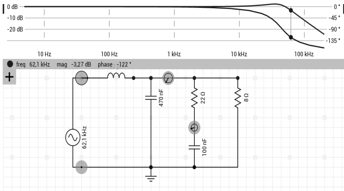
Obrázok 2.13 Simulácia výstupného LC filtra, cievka 22 \mu H
