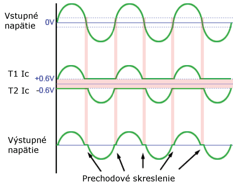
Obrázok 1.1 Prechodové skreslenie [2]
