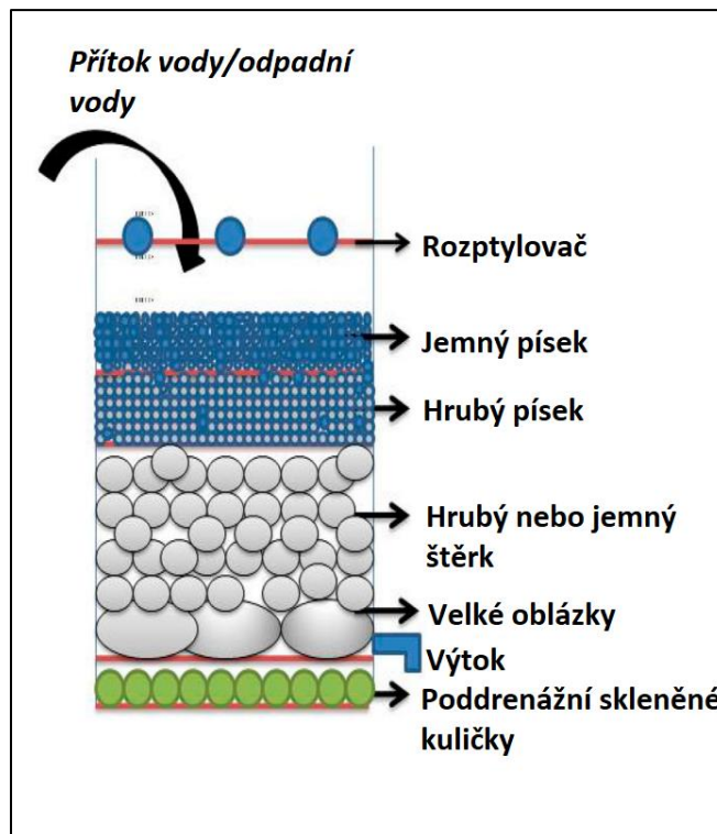
Obrázek 3 Schématické zobrazení pomalé pískové filtrace [10] – přeloženo
