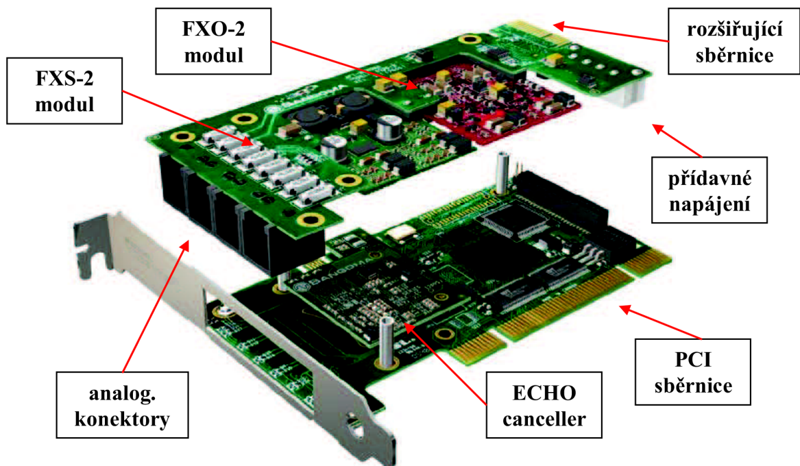
Obr.10: Popis karty Sangoma A200
