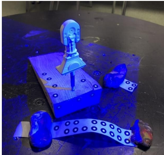
Obr. 19 - Skenovaný díl
