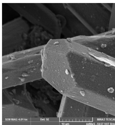
Obr. 48: REM vzorku 3, zvětšeno 4000 x
