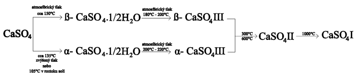
Obr. 1: Schéma dehydratace sádrovce s uvedením všech forem produktů
