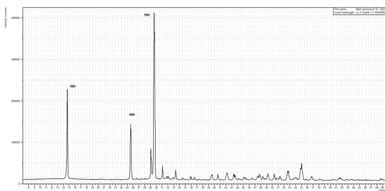
Obr. 68: Rentgenogram vzorku Na25/1 promytý
