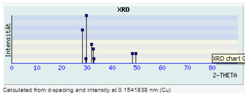
Obr. 6. Rentgenogram Görgeyitu
