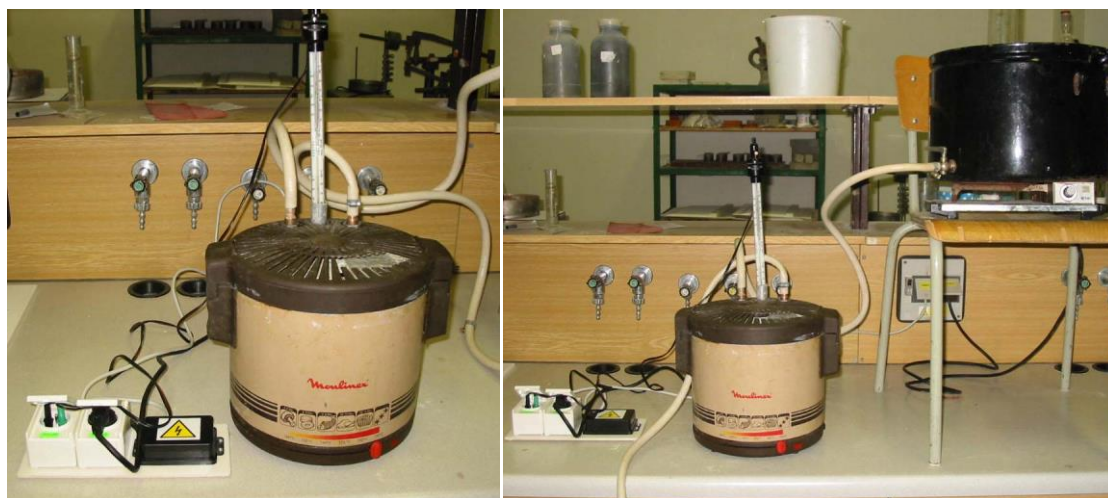
Obr. 15: I. statická verze laboratorního přístroje na výrobu alfa – sádry
