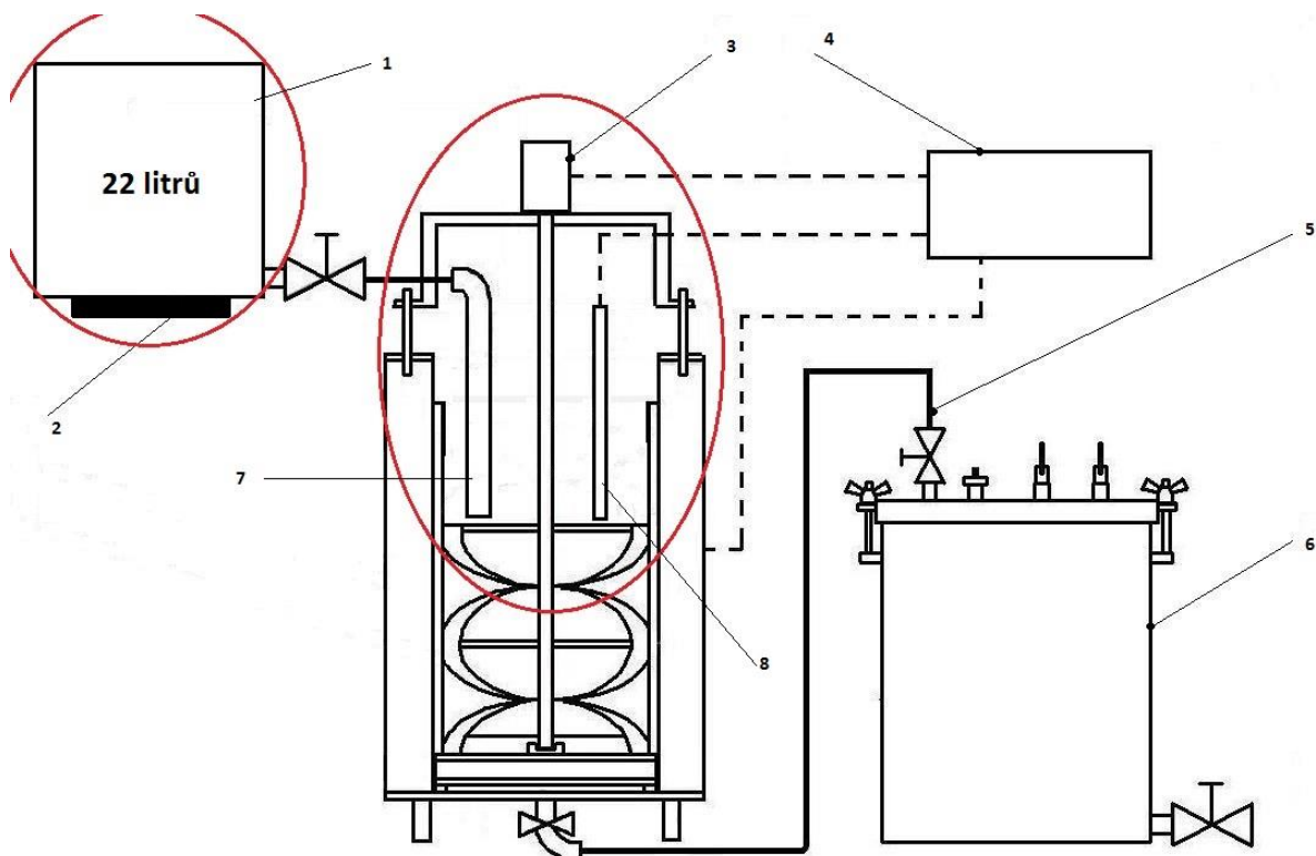
Obr. 49: Dehydratační aparatura po inovaci
