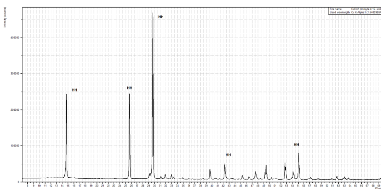
Obr. 64: Rentgenogram vzorku Ca32/2 promytý
