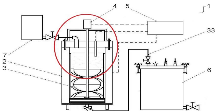
Obr. 29.: Schéma celkové zařízení v původním stav
