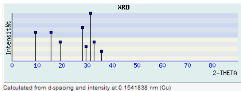
Obr. 12: Rentgenogram Syngenitu
