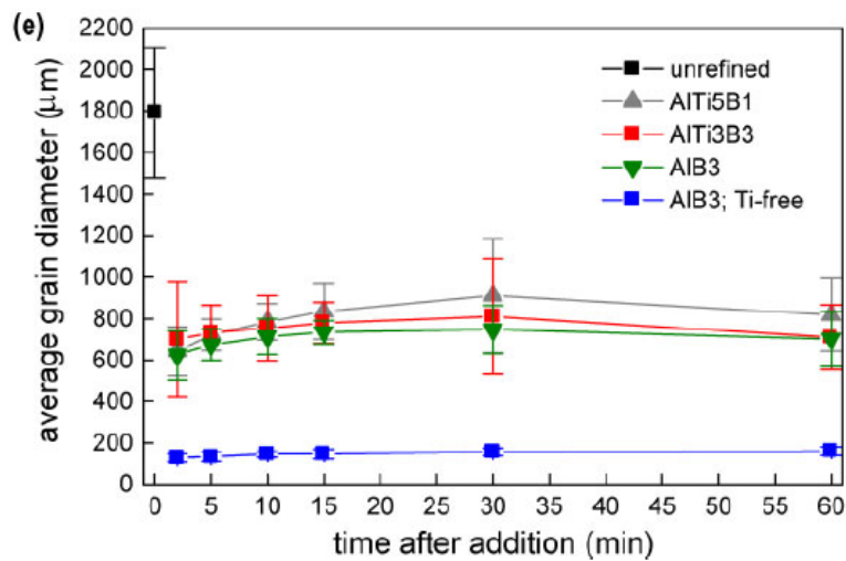
Obrázek 4.2: (a)AlTi5B1, (b)AlTi3B3, (c)AlB3 predzliatina na zjemnenie zrna použitá s komerčnou zliatinou AlSi11Cu, (d)AlB3 predzliatina použitá so zliatinou AlSi11Cu so sniženým obsahom titánu, (e)graf závislosti veľkosti zrna od doby pridania predzliatiny. [14]
