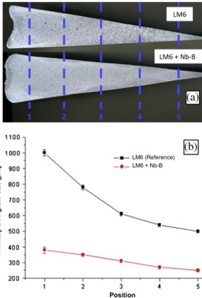
Obrázek 4.3: Vliv rýchlosti ochladzovania na veľkosť zrna. Kuželovitý tvar odliatku zaistil postupnú zmenu rýchlosti ochladzovania po celej dĺžke ochladzovania. [15]
