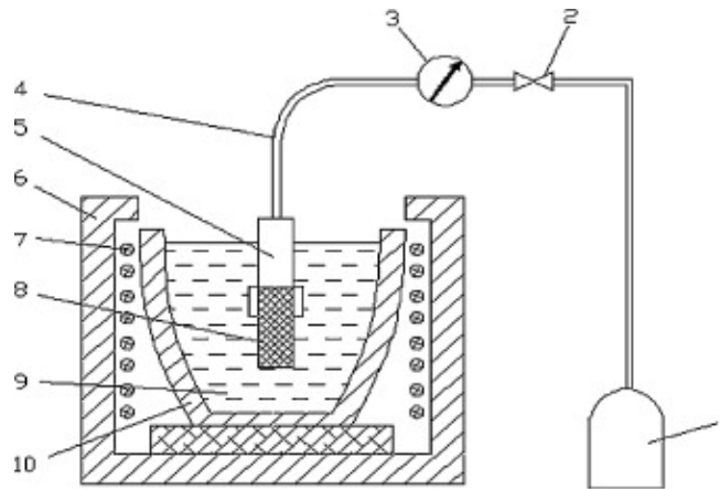
Obrázek 5.4: Schéma vákuového vysávača. 1 - Vákuová pumpa, 2 - ventil, 3 - vakuometer, 4 - trubica spájajúca vákuovú pumpu so sacou hlavicom, 5 - spoj, 6 - pec, 7 - ohrievací element, 8 - vysávacia hlavica, 9 - tavenina, 10 - kelímok, [7]
