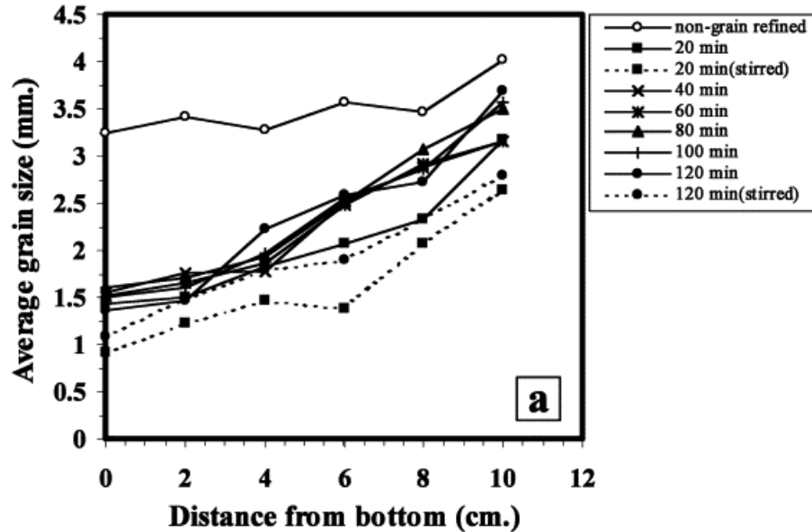
Obrázek 4.1: Graf ukazujúci závislosť veľkosti zrna od vzdialenosti od dna odliatku rôznych vzoriek odliatych pri rôznych podmienkach. Vzorky boli odliate pri rôznych časoch výdrže v roztavenom stave. [13]
