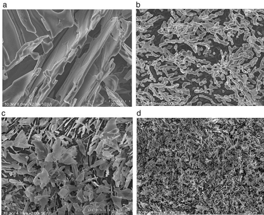
Obrázek 4.5: Mikroštruktúra eutektika pri rôznych rýchlostiach ochladzovania. a)Grafitový kelímok, bez modifikácie, b)Grafitový kelímok, modifikácia stronciom 54ppm, c)Oceľová forma, bez modifikácie, d)Oceľová forma, modifikácia stronciom 54ppm [11]
