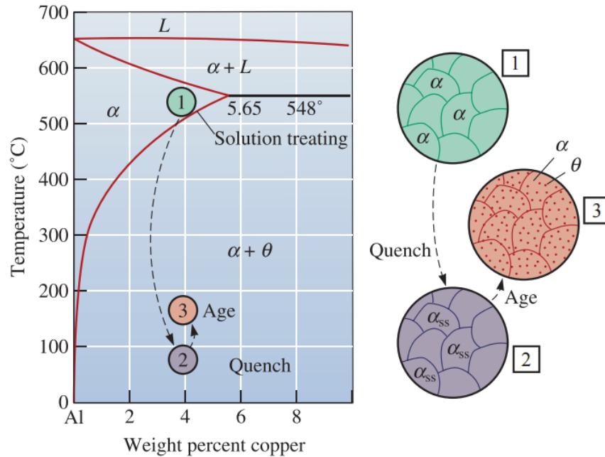
Obrázek 6.1: Výsek binárneho diagramu Al-Cu znázorňujúci proces vytvrdzovania. 1) Rekrystalické žihanie; 2) Rýchle ochladenie; 3) Stárnutie [24]
