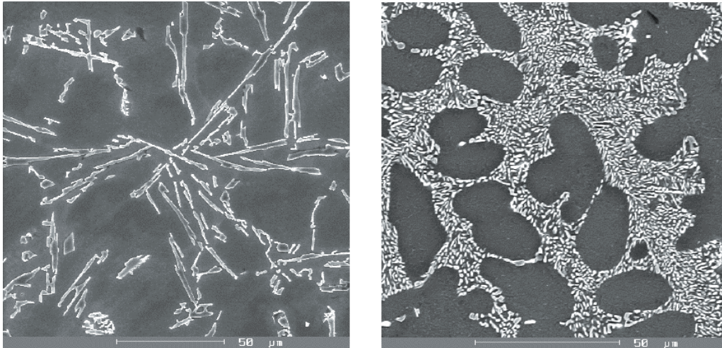
Obrázek 4.4: V ľavo nemodifikované eutektikum, v pravo modifikované eutektikum. [1]
