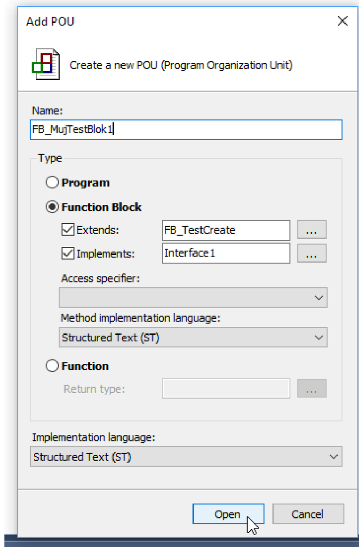
Obr. 19: Add POU přidání názvu
