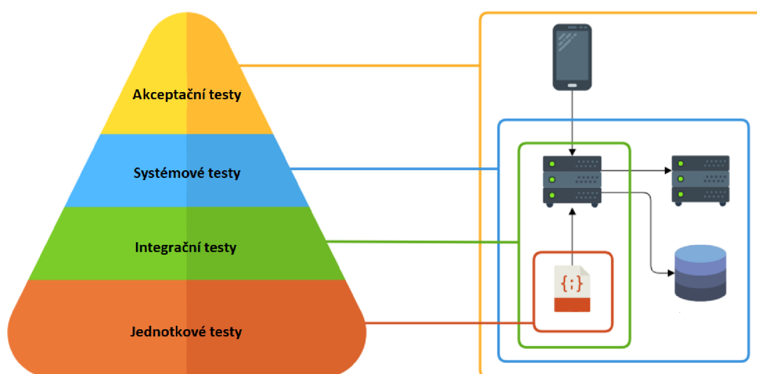
Obr. 1: Úrovně testů [25]
